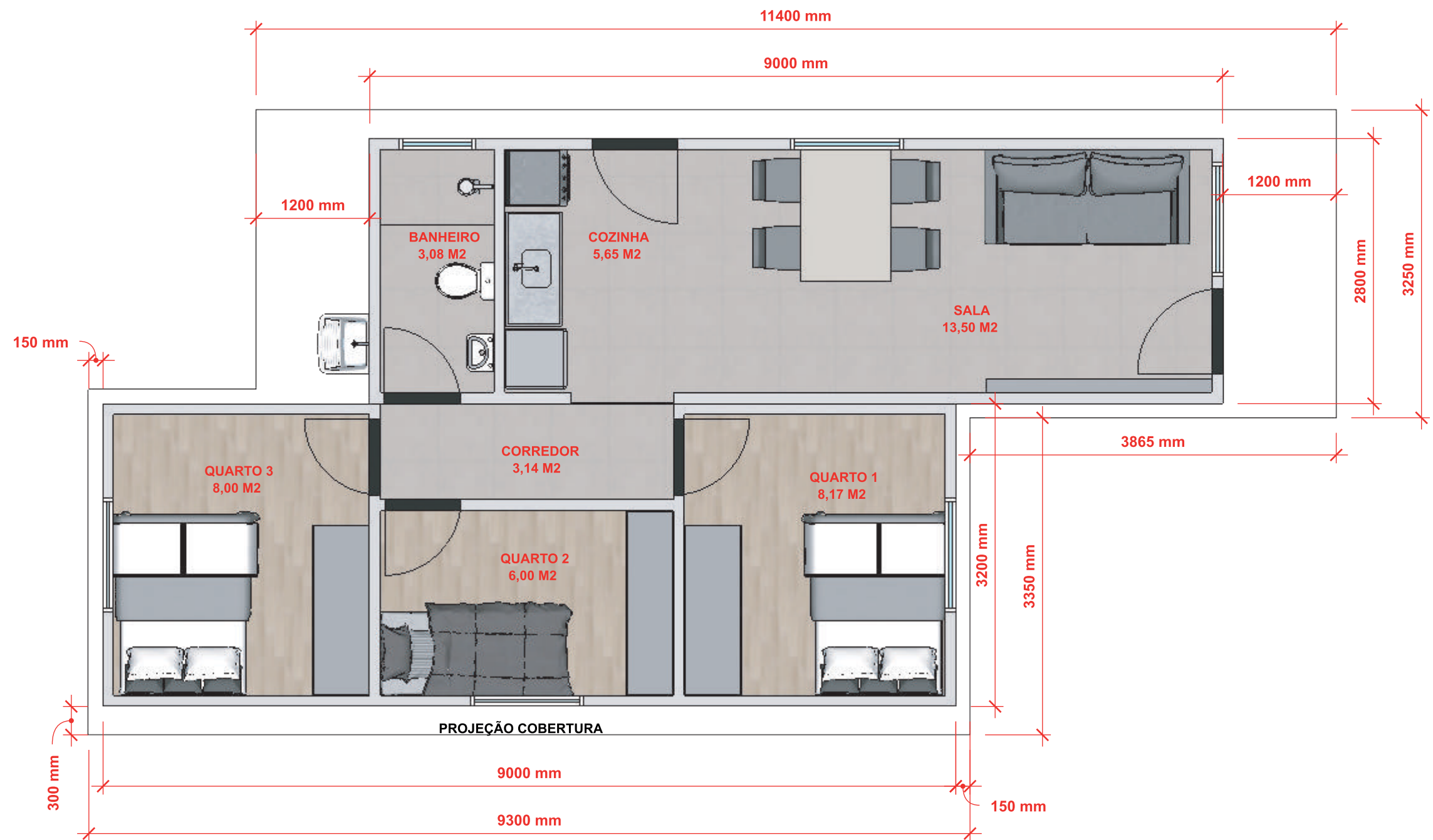
01 PLANTA BAIXA 1:50
