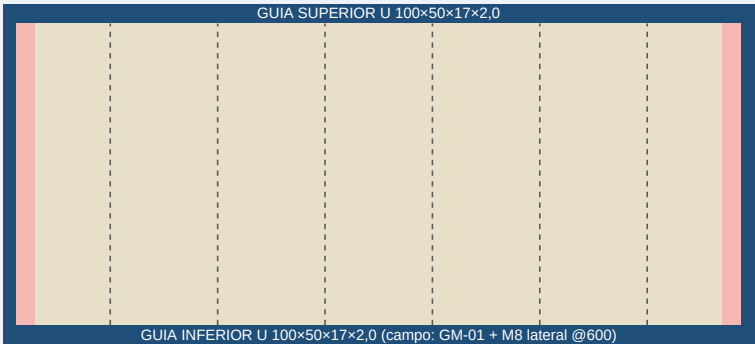
CROQUI ESQUEMÁTICO — posições exatas de vãos e MEP: GABARITO DE COORDENADAS (IFC R14 / abas 01-04-05) — fonte única
