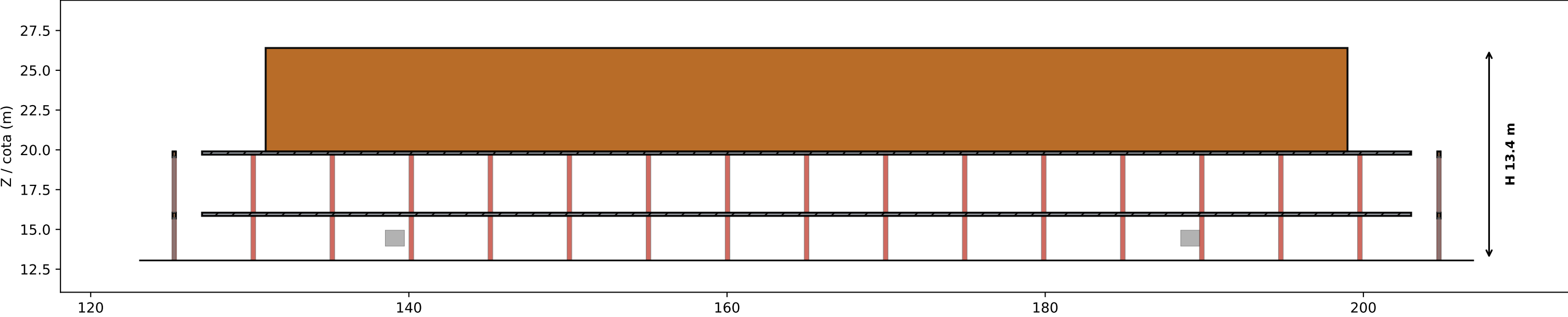
HVG BRUMADINHO - BLOCO PRINCIPAL - CORTE LONGITUDINAL (Y=245) cotas em m
