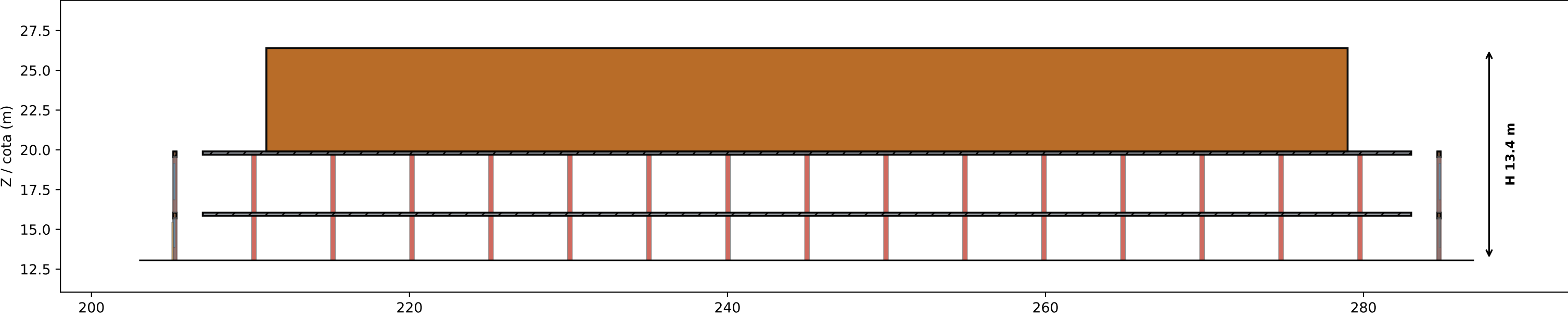
HVG BRUMADINHO - BLOCO PRINCIPAL - CORTE TRANSVERSAL (X=165) cotas em m
