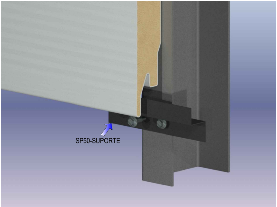
DET. TÍPICO SUPORTE SAÍDA DE MONTAGEM
