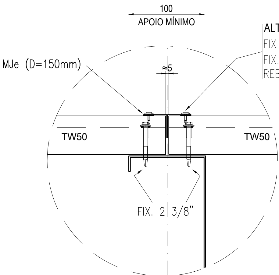
DETALHE APOIO MÍNIMO PARA FIXAÇÃO DE DOIS PAINELIS (CHEGADA DE TOPO) ESC.1:7,5
