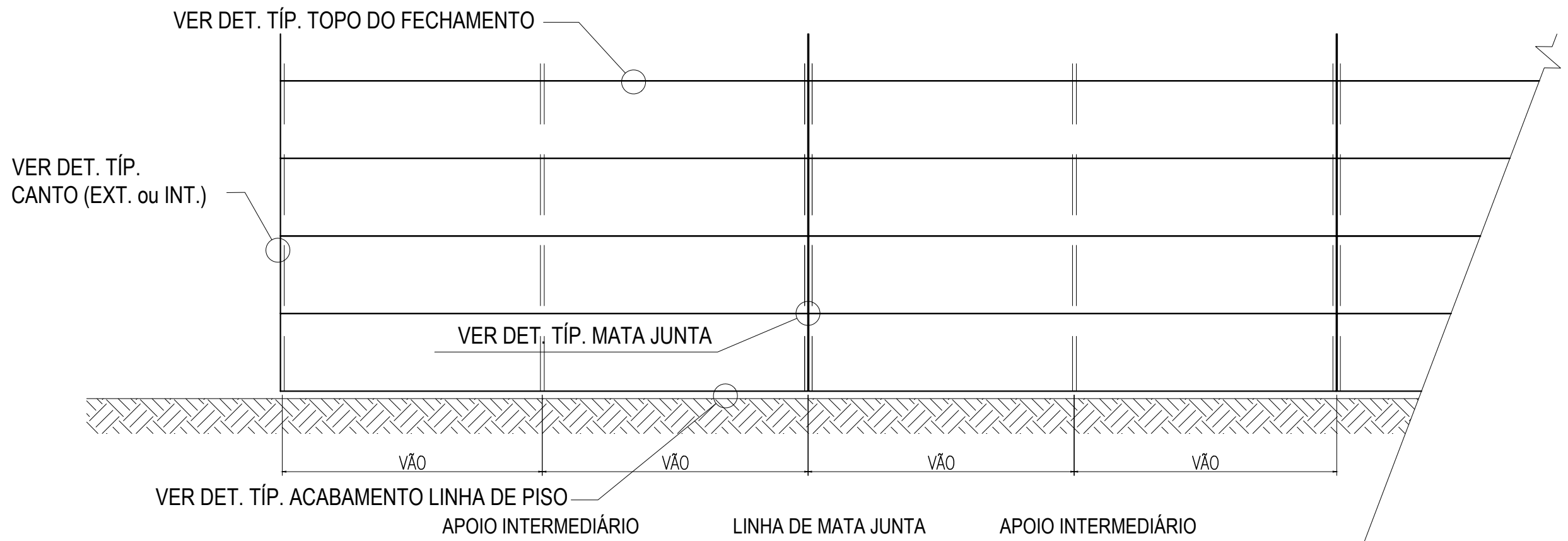
ELEVAÇÃO FECH. HORIZONTAL PAINEL TW50-MN
