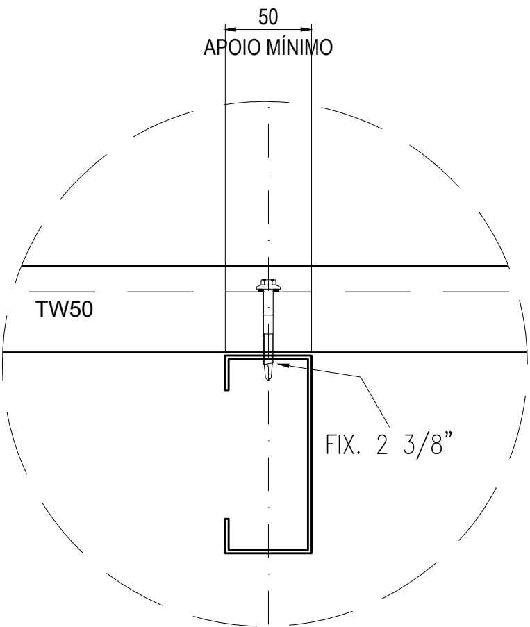
DETALHE APOIO MÍNIMO PARA FIXAÇÃO DE UM PAINEL ESC.1:7,5
