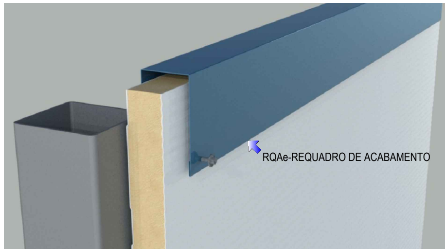
DET. TÍP. TOPO DO FECHAMENTO
