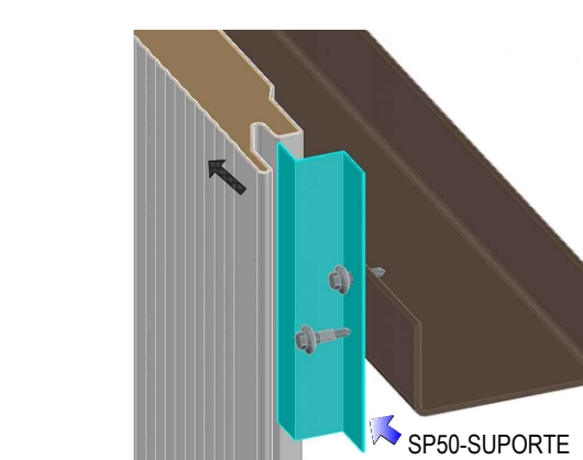
DET. TÍPICO SUPORTE SAÍDA DE MONTAGEM
