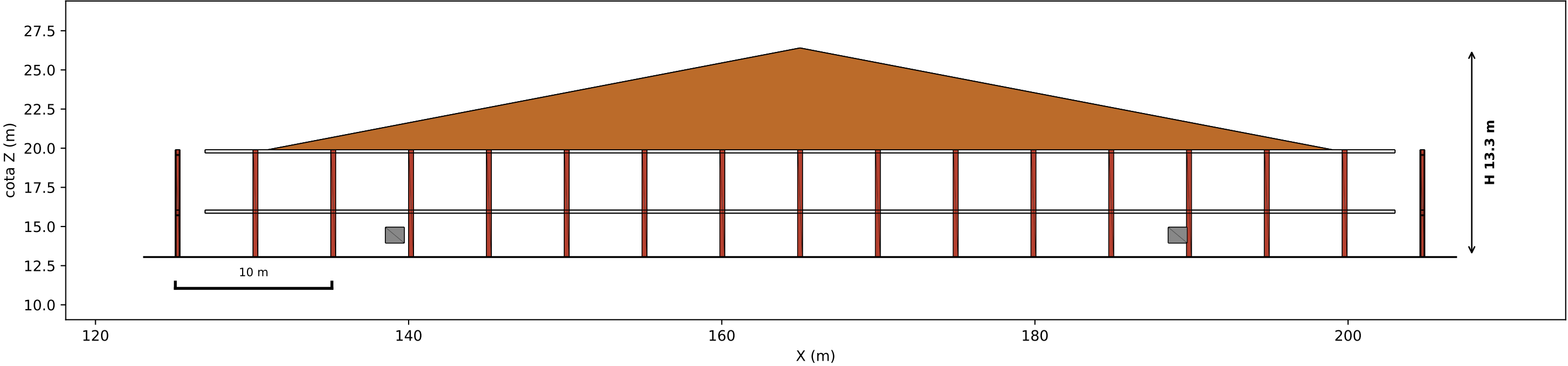
BLOCO PRINCIPAL - CORTE LONGITUDINAL (Y=245)
