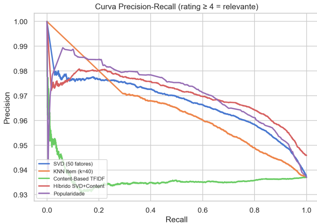
Figura 9: Curva Precision-Recall (rating ≥ 4 = relevante).
