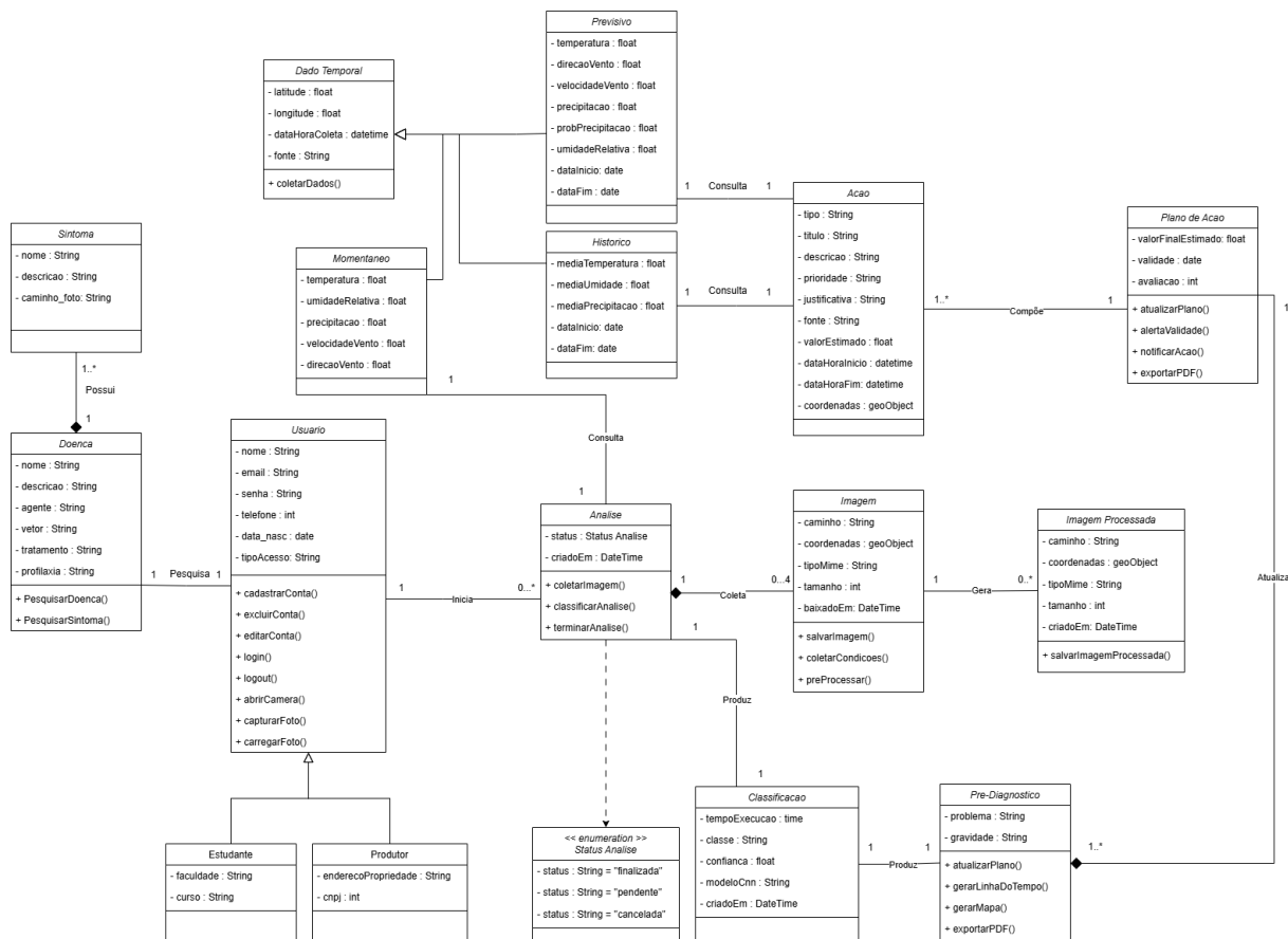
Figura 5: Diagrama de Classes do Sistema
