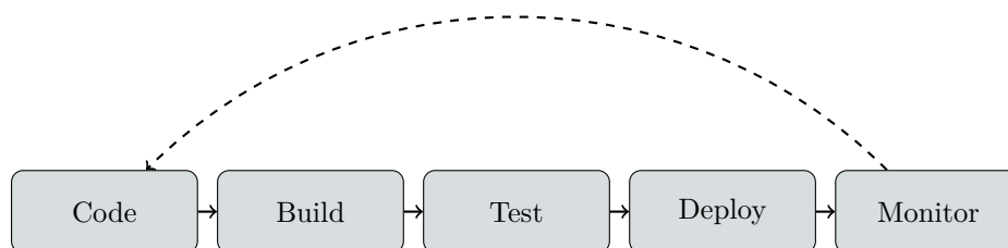
Figura 7: Pipeline CI/CD
