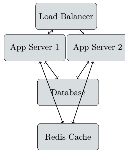
Figura 7: Arquitetura de Deployment
