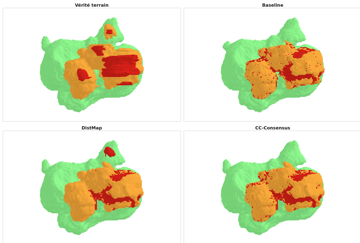
Figure 7: Figure 7 — Cas C6 (patient BraTS-GLI-00388-000) : mode « casse » quasi éteint en régime officiel : F < \min(B, D) pour seulement 2/1196 (0,2 %), écart maximal 0,0007. Ici la fusion reste juste sous le pire parent ( 0,921 contre 0,923/0,922). Mesuré avec la même méthode sur les mêmes 1196 patients, ce mode valait 47/1196 (3,9 %) sur les prédictions brutes, avant le nettoyage officiel.
