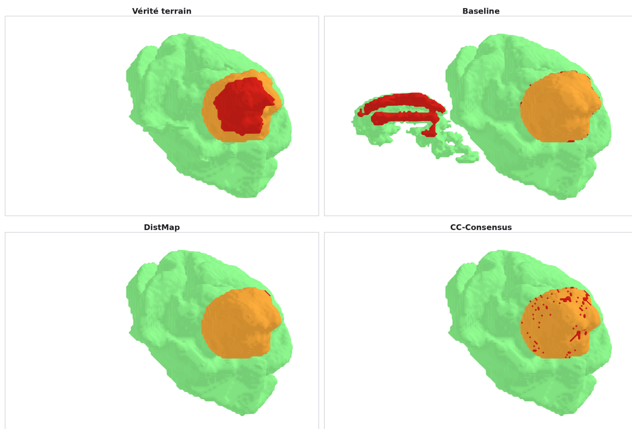
Figure 3: Figure 3 — Cas C2 (patient BraTS-GLI-01094-000) : le filtre confirme DistMap (1183/1196, 98,9 % des patients — mode majoritaire en régime officiel). Baseline sous-segmente la tumeur (0,643 ; WT \approx 0,49, HD95 \approx 188 mm) ; DistMap est précis (0,968, HD95 1,0 mm) et ne génère aucune composante fallacieuse : après le nettoyage officiel, toutes ses composantes sont corroborées par Baseline, le veto ne retire rien ( F = D = 0,968 ).
