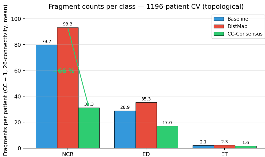
Figure 1: Figure 1 — Comptage moyen de fragments par patient (composantes connexes non-principales, 26-connectivité, sans seuil de taille) pour chaque classe × variante, sur les 1196 patients de la CV 5-fold. DistMap inflat le nombre de fragments NCR de +17 % par rapport à Baseline ; le filtre CC-consensus le ramène à 31,3 — une réduction de 66 % par rapport à DistMap (Wilcoxon p < 10^{-189} ).
