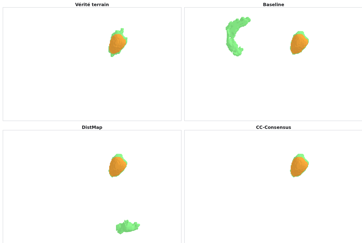
Figure 6: Figure 6 — Cas C5 (patient BraTS-GLI-00733-001) : synergie, \mathbf{F} > \max(\mathbf{B}, \mathbf{D}) (2/1196, 0,2 %). Baseline (0,751) et DistMap (0,805) perdent tous deux une grande partie de la tumeur entière (Dice WT \approx 0,32/0,48 , HD95 \approx 250/188 mm) ; le CC-Consensus restaure le contour WT (0,955, HD95 1,4 mm) et atteint 0,964 — strictement supérieur aux deux parents .
