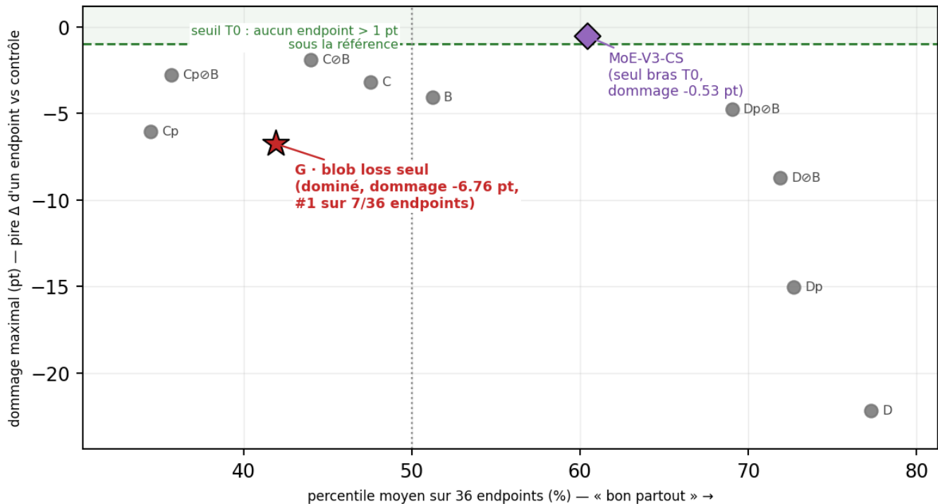
Figure 3: F3 — G dans le classement de polyvalence
