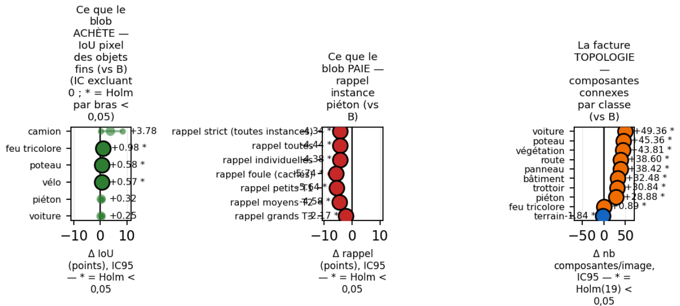
Figure 2: F2 — Le trade-off mesuré
