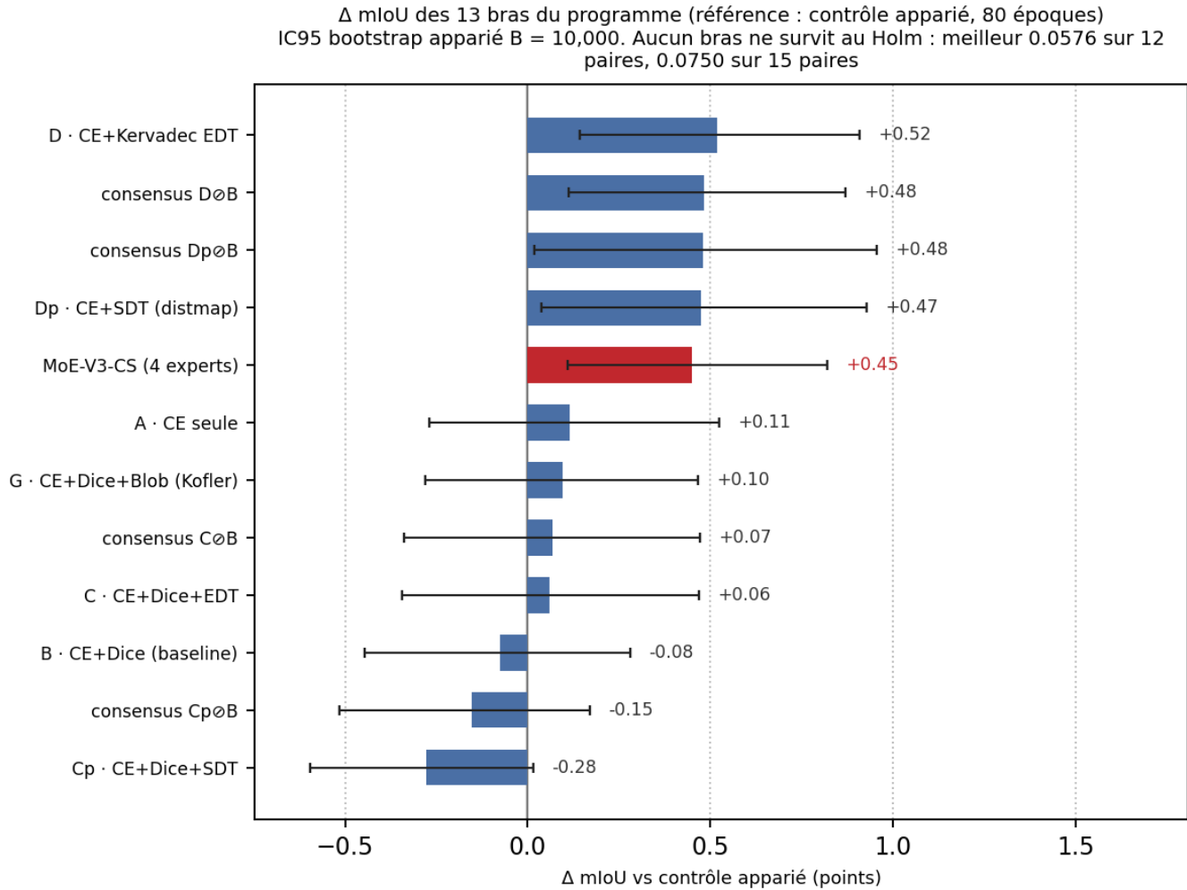
Figure 1: F1 — \Delta mIoU des 13 bras contre le contrôle apparié, avec IC95
