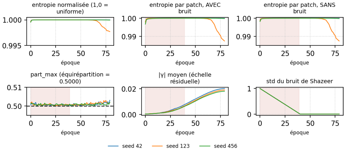
Figure 2: F2 — Routage sur 80 époques × 3 seeds : frac, entropies, \gamma
