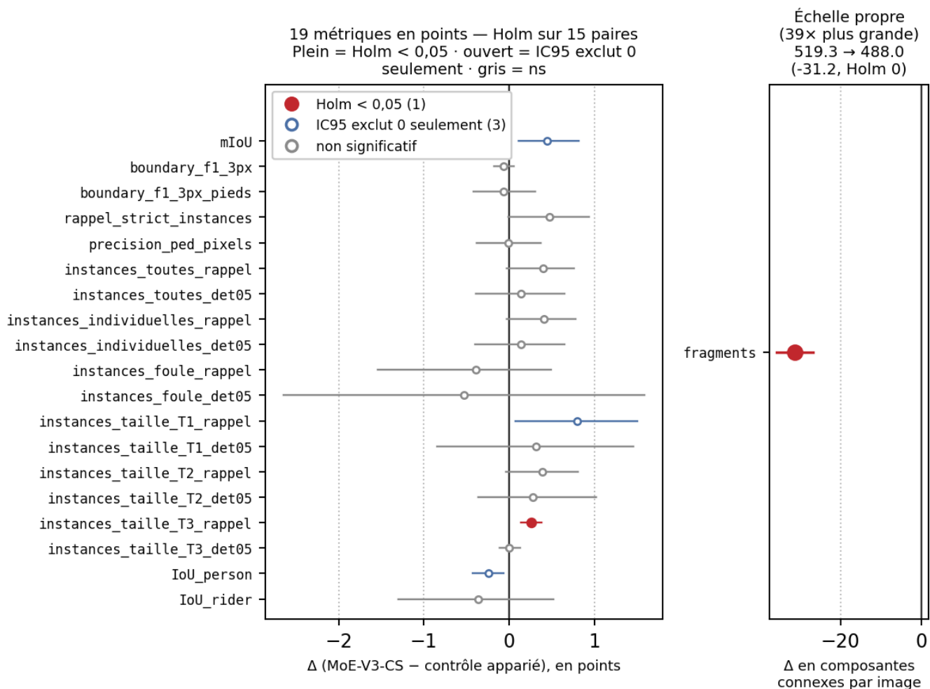
Figure 3: F3 — Forest plot des métriques métier, deux panneaux à unités distinctes. \Delta (MoE – contrôle) des métriques métier avec IC95 : les deux panneaux portent des unités distinctes — les 19 métriques en points sur un axe, fragments ( \Delta -31,2 composantes par image) sur le sien — car les tracer ensemble compresserait les métriques en points d'un facteur \approx 39 en une bande illisible.
