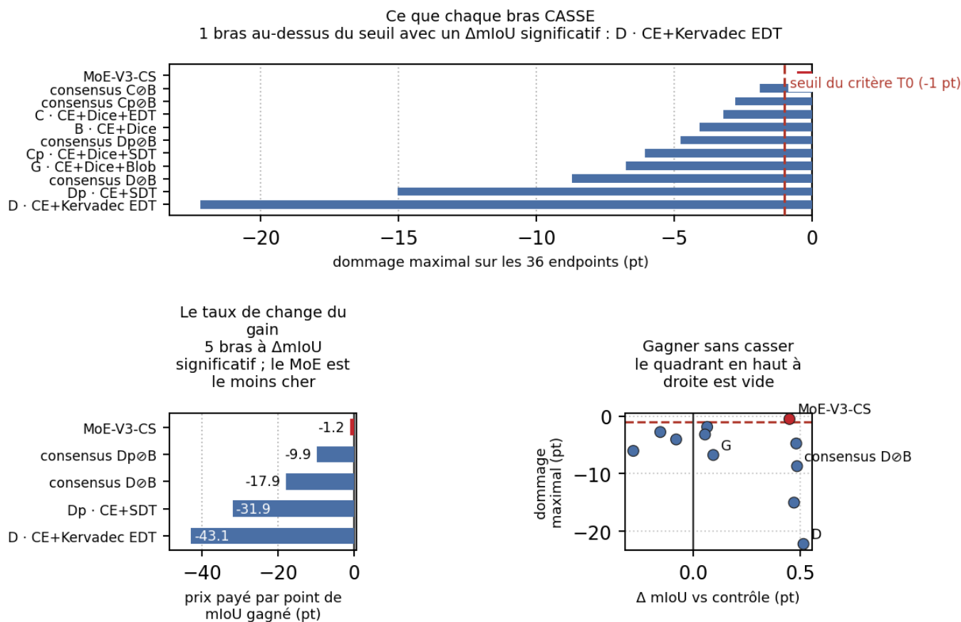
Figure 5: F4 — Polyvalence : 3 panneaux (dommage maximal, prix payé par point de mIoU, gagner sans casser)
