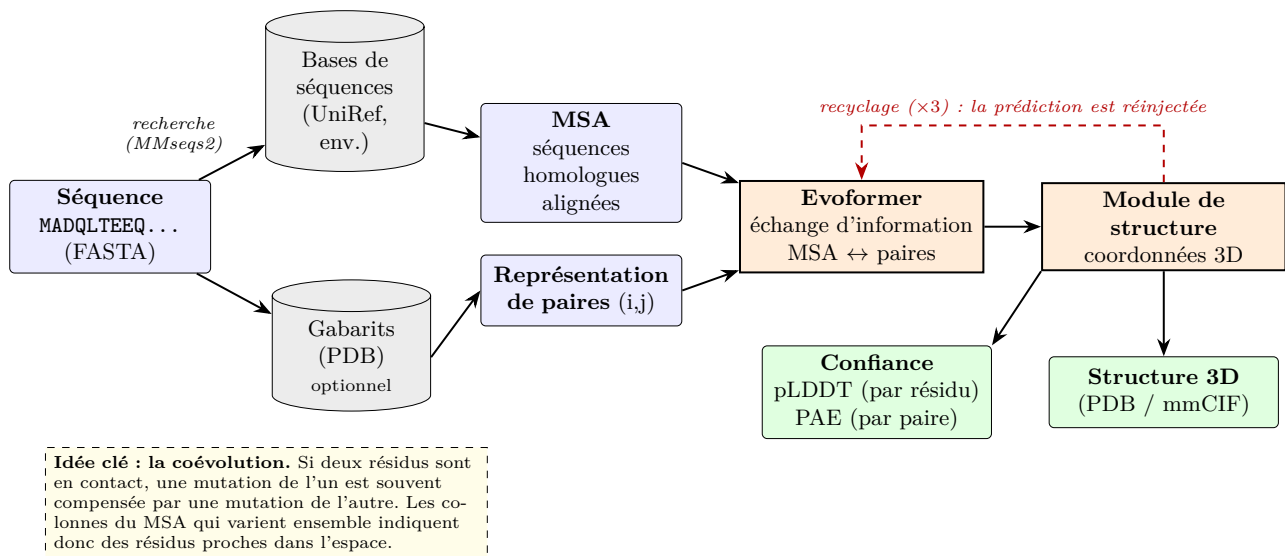
FIGURE 1 – Schéma du fonctionnement général d'AlphaFold2 (réalisation personnelle, d'après [8, 6]).
