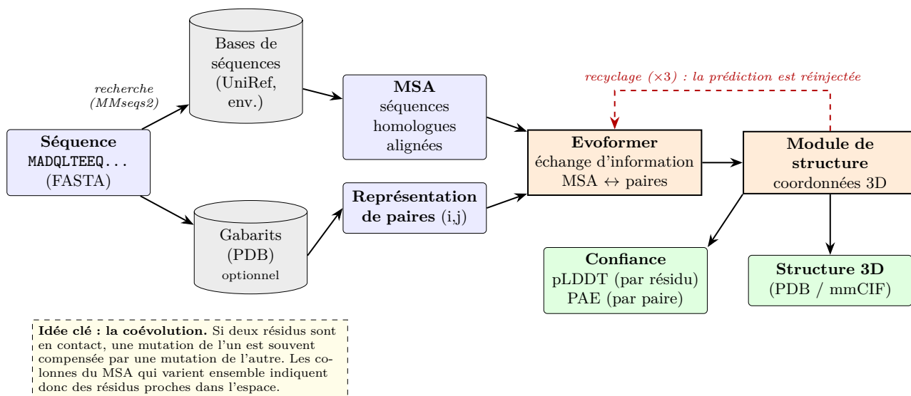
FIGURE 1 – Schéma du fonctionnement général d'AlphaFold2 (réalisation personnelle, d'après [11, 6]).
