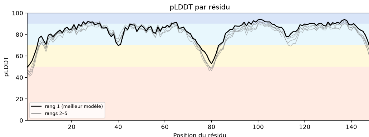
FIGURE 4 – pLDDT par résidu du meilleur modèle (noir) et des 4 autres (gris). Fonds colorés : classes de confiance.
