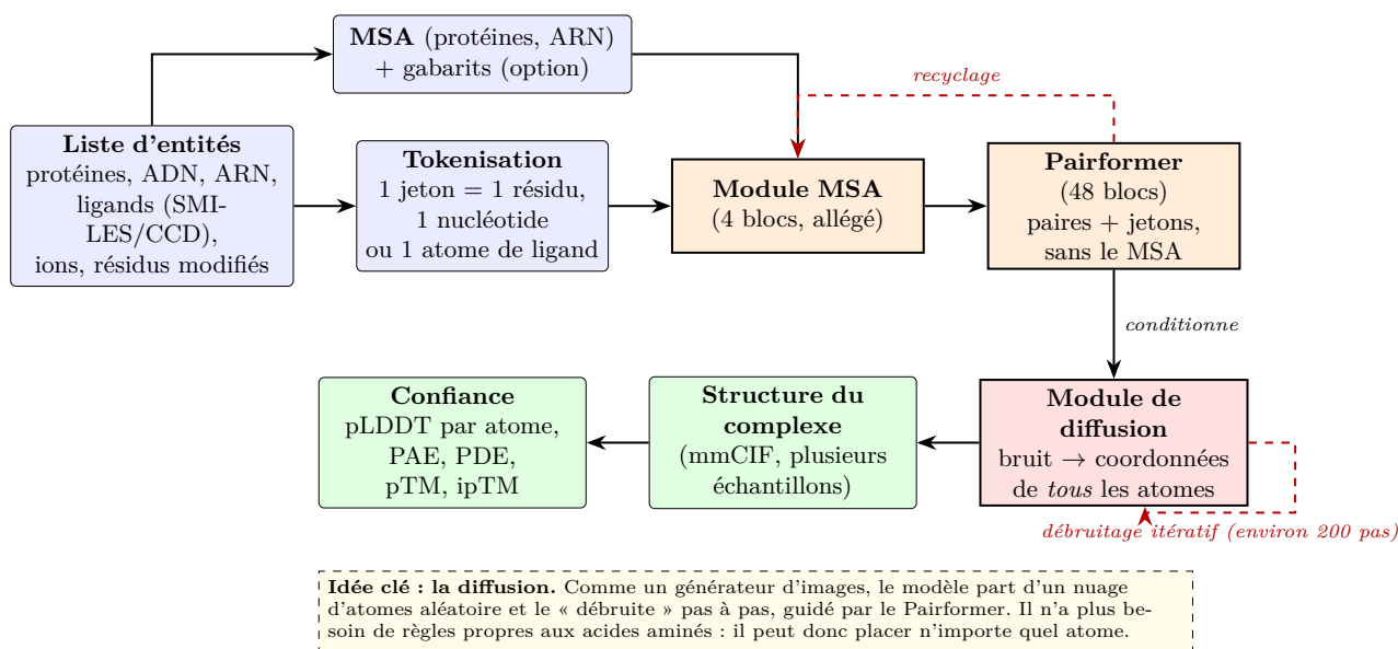
FIGURE 2 – Schéma du fonctionnement général d'AlphaFold3 (réalisation personnelle, d'après [1]).
