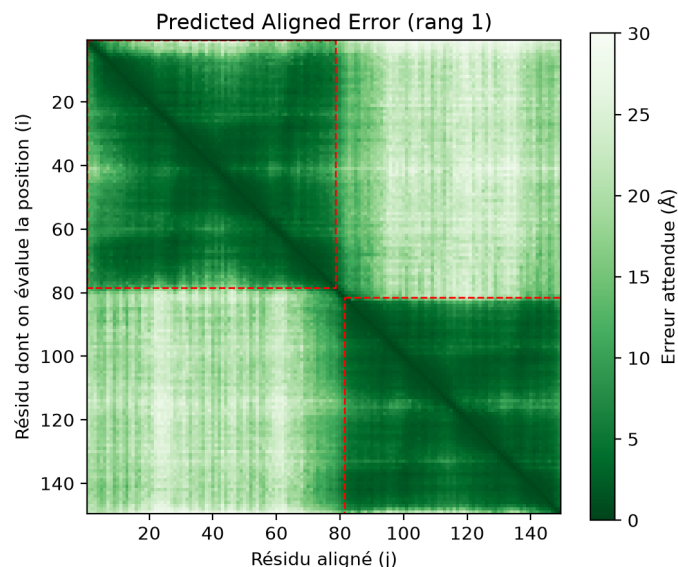
FIGURE 5 – Matrice PAE du meilleur modèle. Cadres rouges : lobe N (1–78) et lobe C (82–149).
