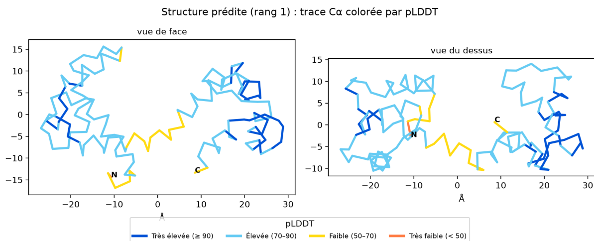
FIGURE 3 – Trace C \alpha du meilleur modèle, colorée par pLDDT (produite par scripts/analyse.py ). Elle peut aussi être visualisée en 3D en déposant le fichier PDB sur https://molstar.org/viewer/ .
