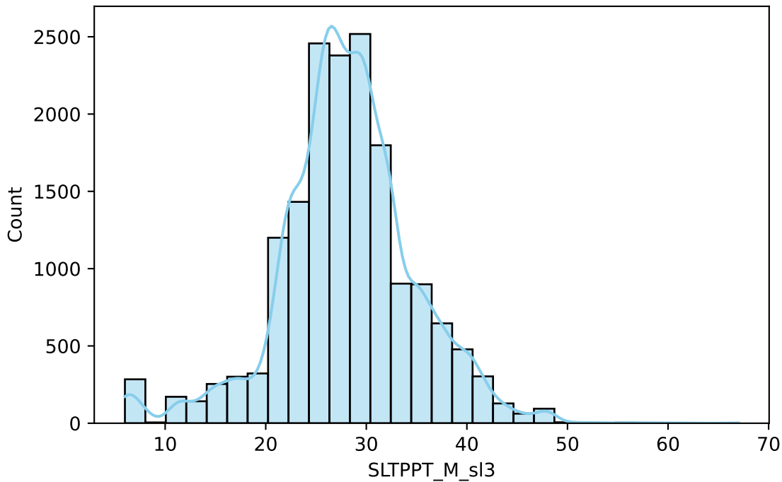
SLTPPT_M_sl3
