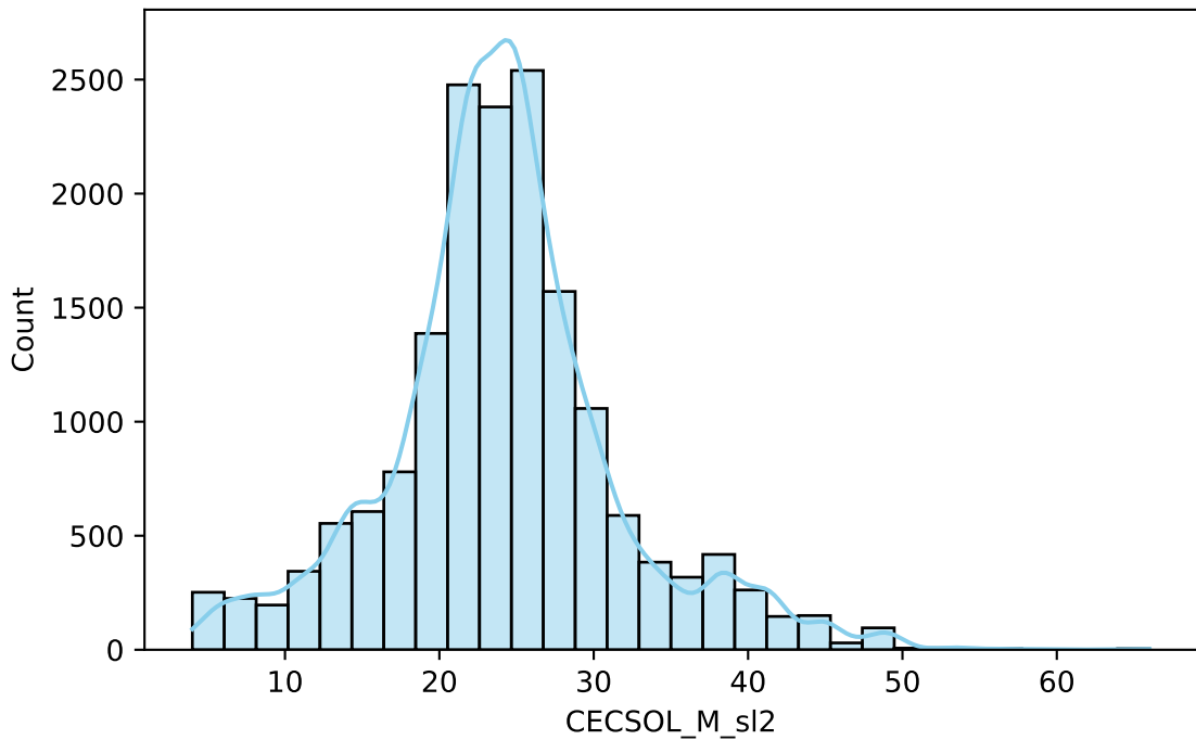
CECSOL_M_sl2
