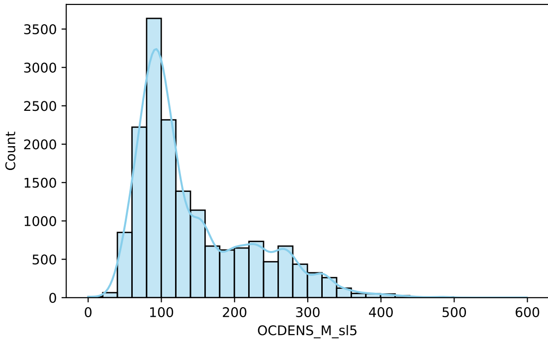
OCDENS_M_sl5
