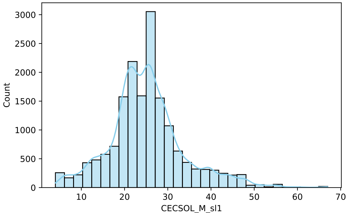
CECSOL_M_sl1
