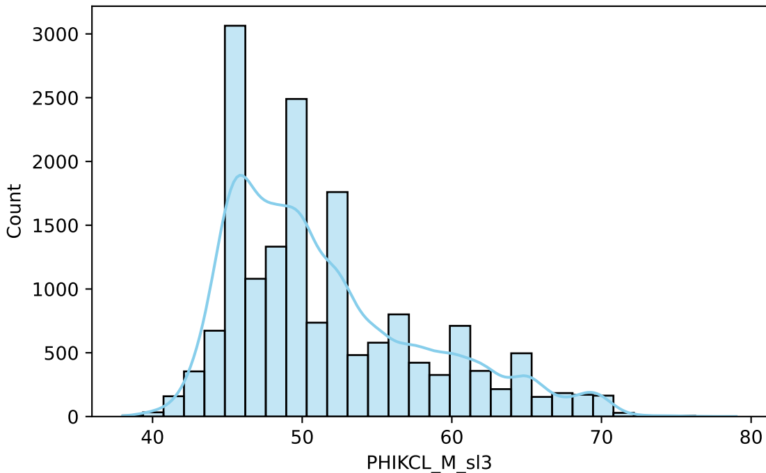
PHIKCL_M_sl3
