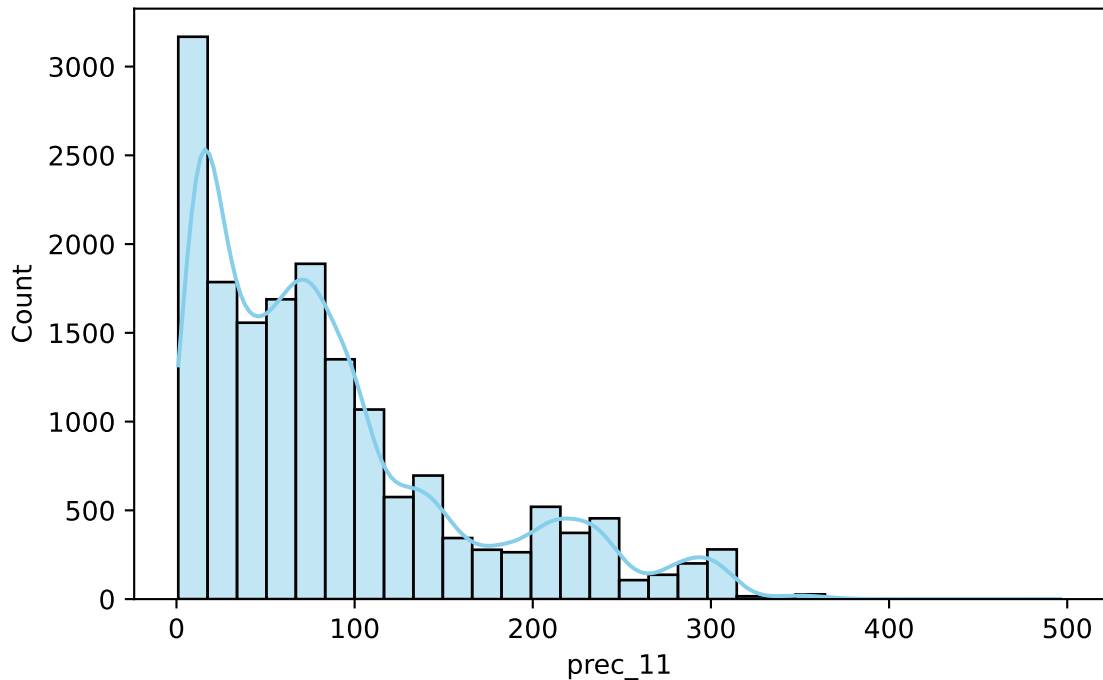
prec_11
