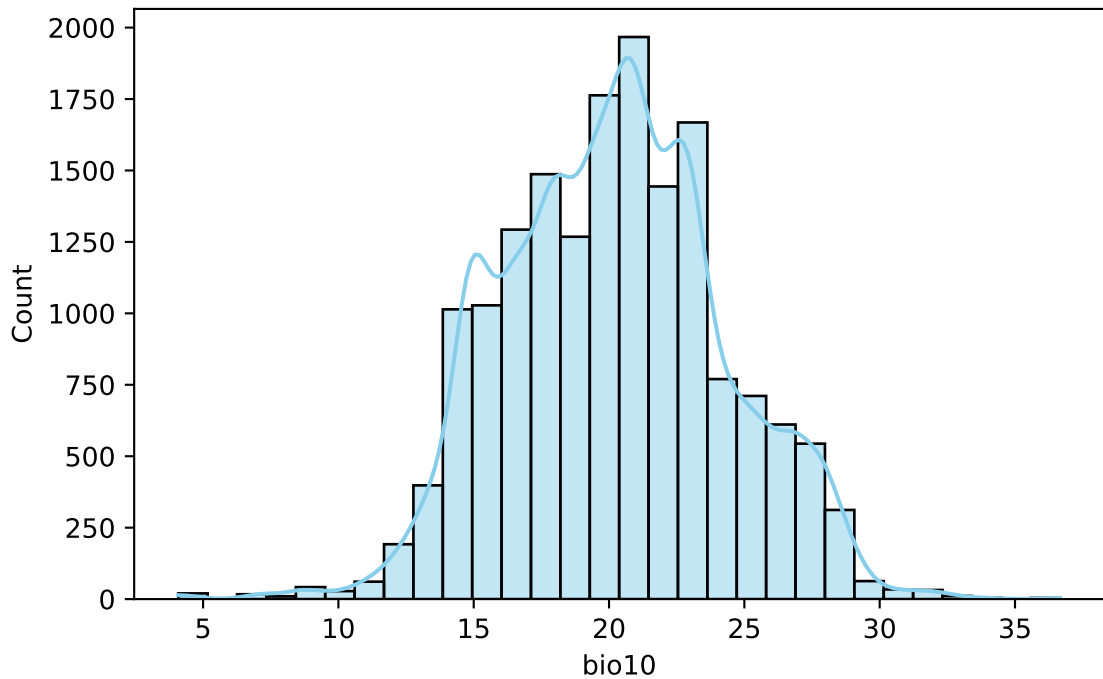
bio10
