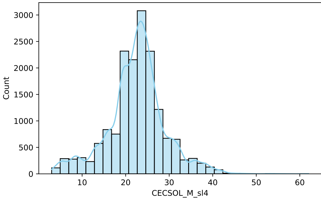
CECSOL_M_sl4
