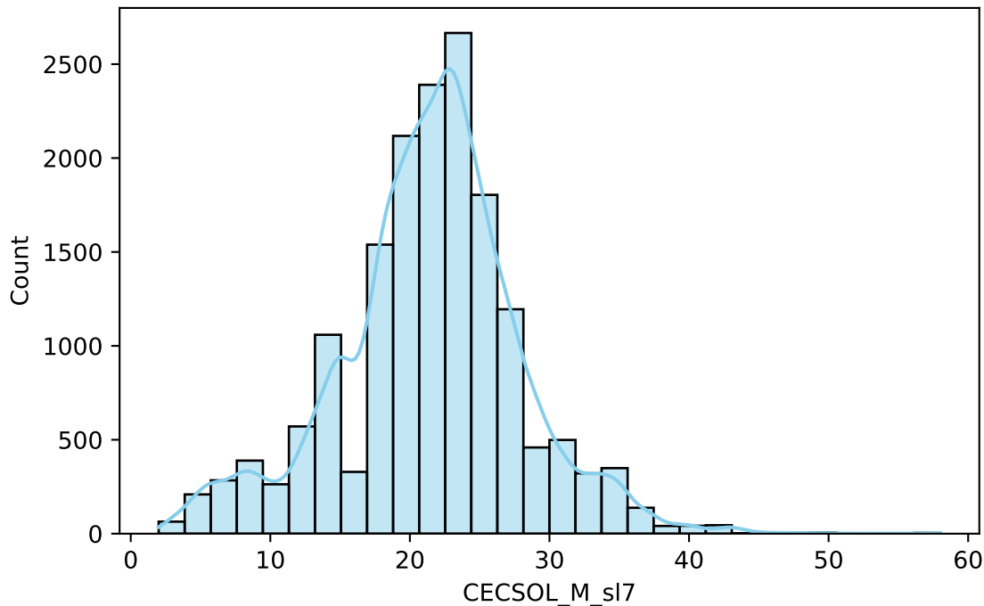
CECSOL_M_sl7
