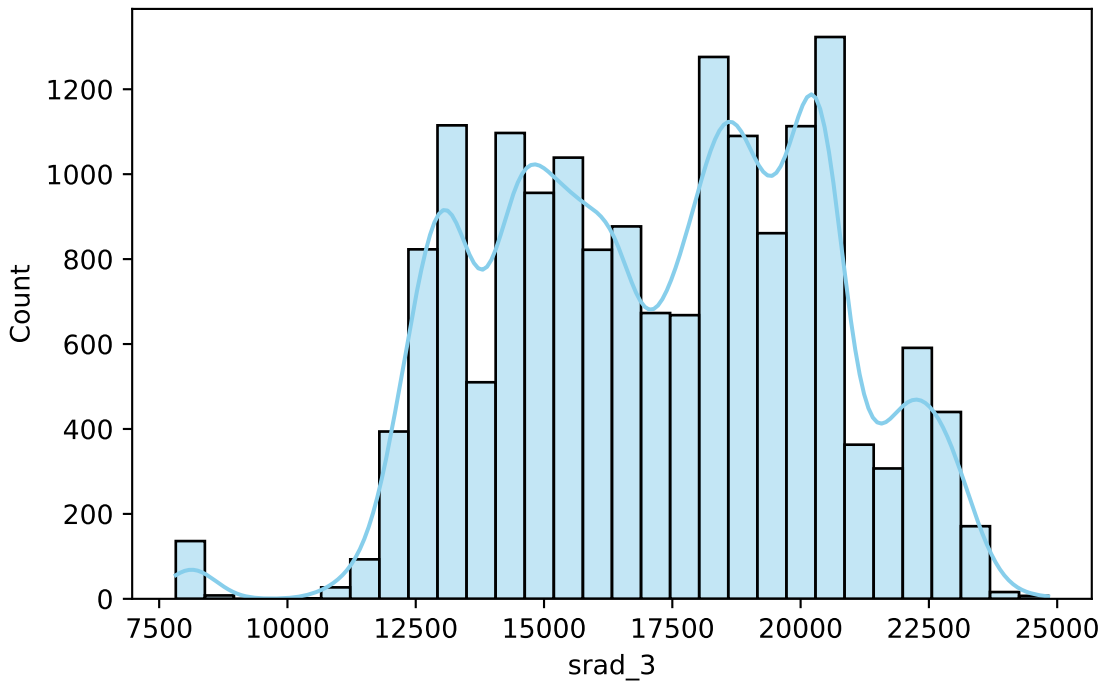
srad_3
