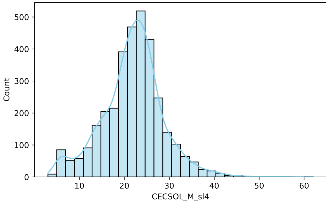
CECSOL_M_sl4
