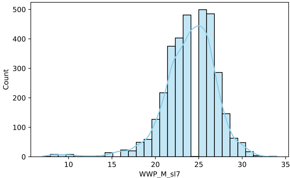
WWP_M_sl7
