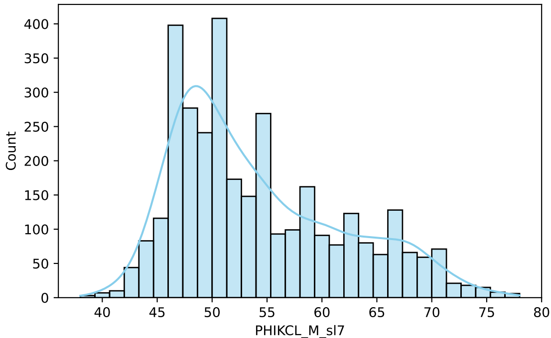
PHIKCL_M_sl7
