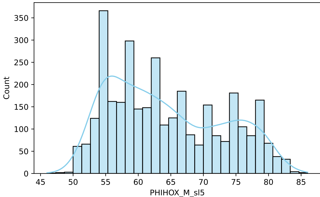
PHIHOX_M_sl5
