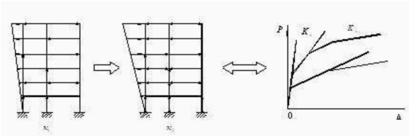
图3.2 非线性构形状态转移过程示意图
