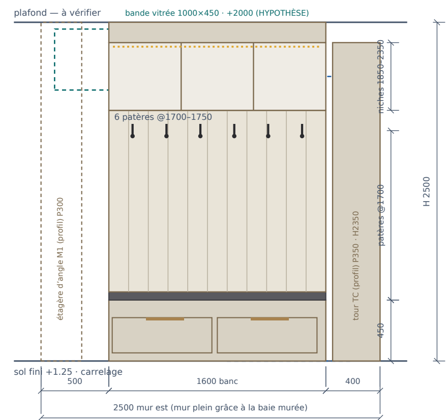
ÉLÉVATION B1 · ≈ 1:28 @ A3 — banc 1600 · 2 tiroirs · 6 patères · 3 niches tireté bleu = ancienne baie de porte murée (arrière-plan) · tireté teal = bande vitrée (dans le mur)
