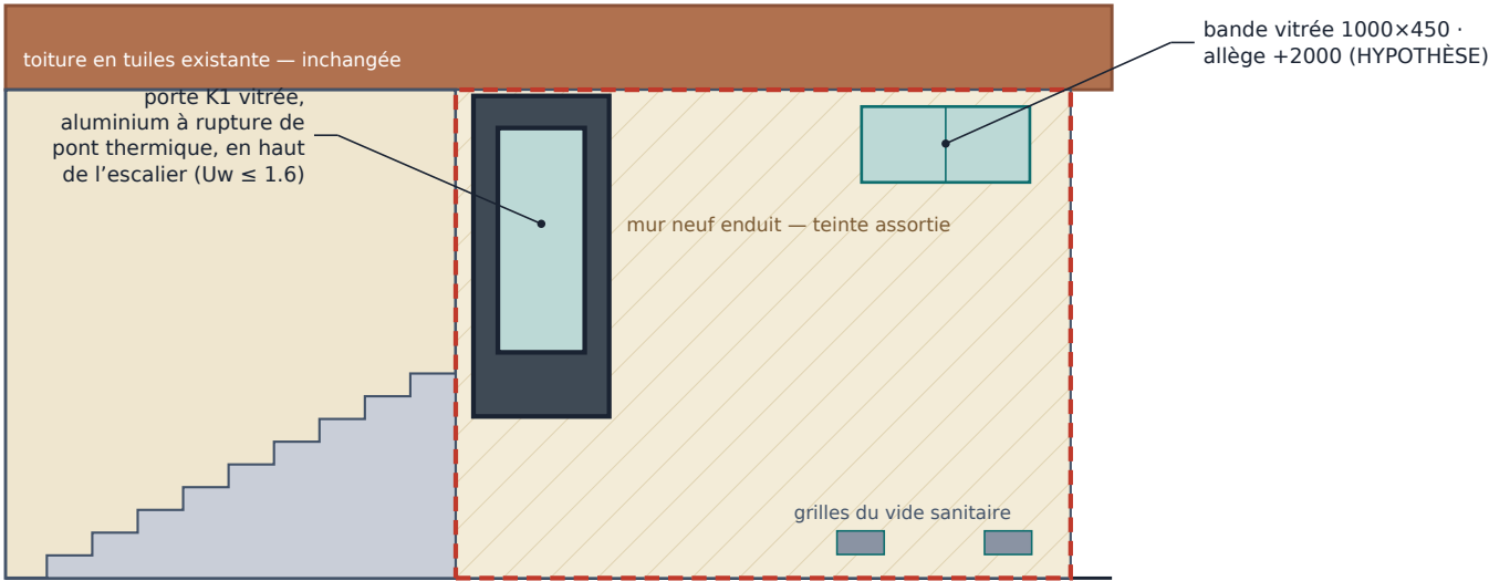
PROJET · façade d’entrée · ≈ 1:60
