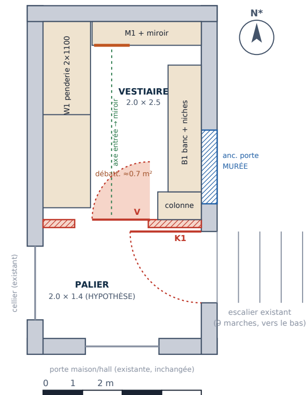
Plan schématique — cotes en mm, nominales. Relevé sur site obligatoire avant toute fabrication.
