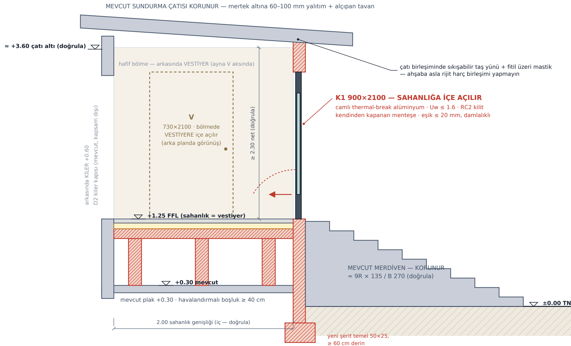
B-B KESİTİ • ÖLÇEK \approx 1:26 @ A3 • sahanlık boyunca kuzeye bakış — K1 kesitte, V bölmede görünüşte
