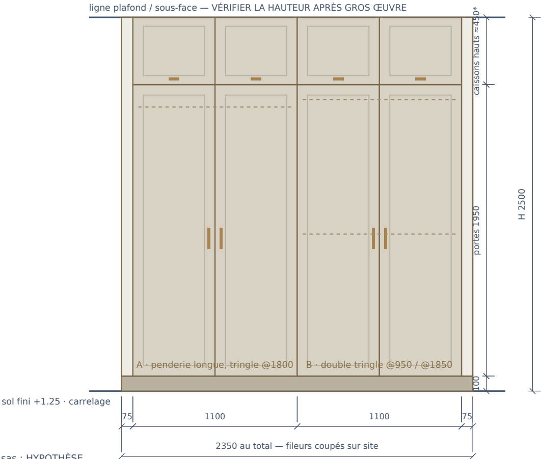
ÉLÉVATION W1 · ≈ 1:26 @ A3 — 2 modules 1100 à double porte · porte 1950 + caisson haut · profondeur 600
