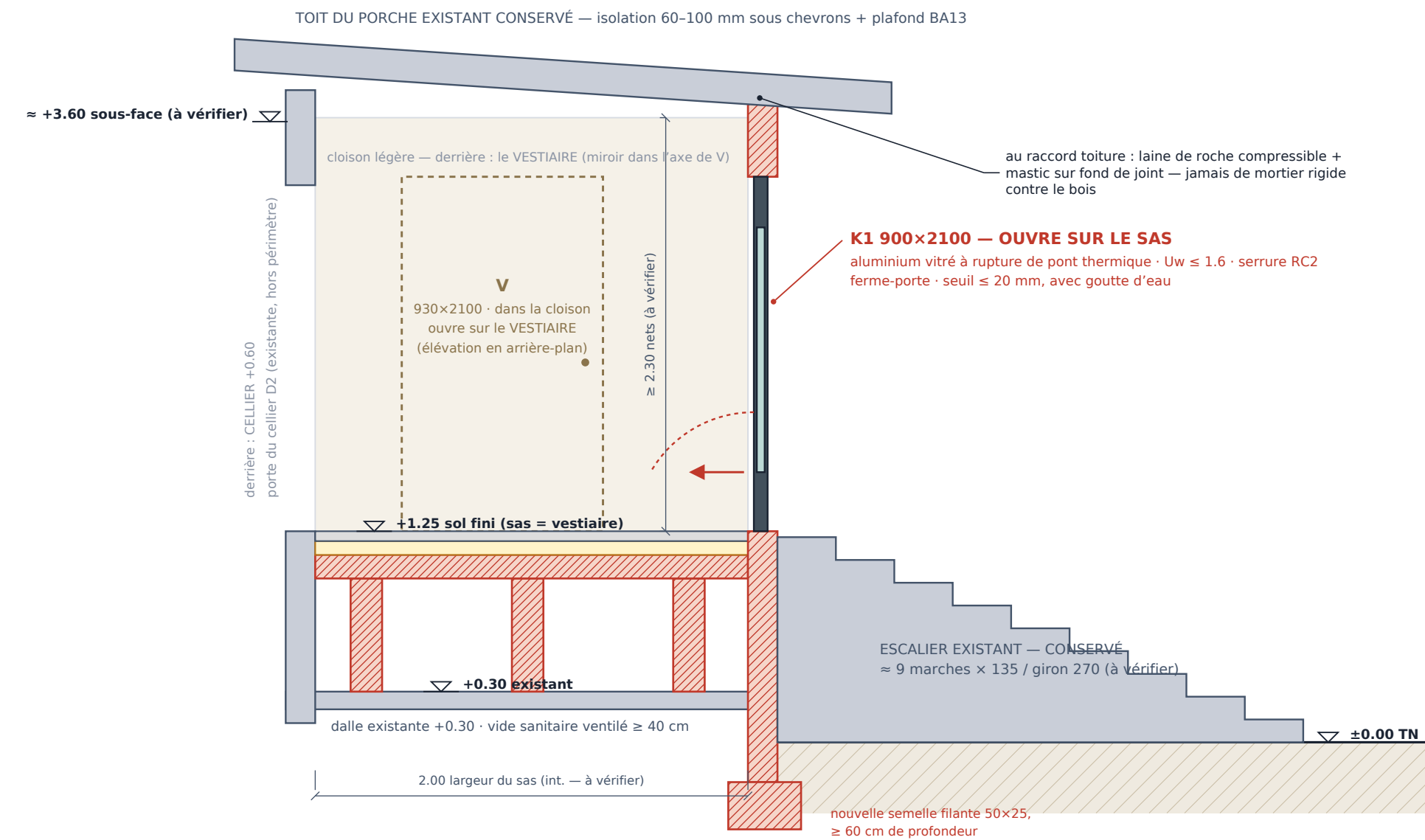
COUPE B-B · ÉCHELLE ≈ 1:26 @ A3 · vue vers le nord le long du sas — K1 en coupe, V en élévation dans la cloison
