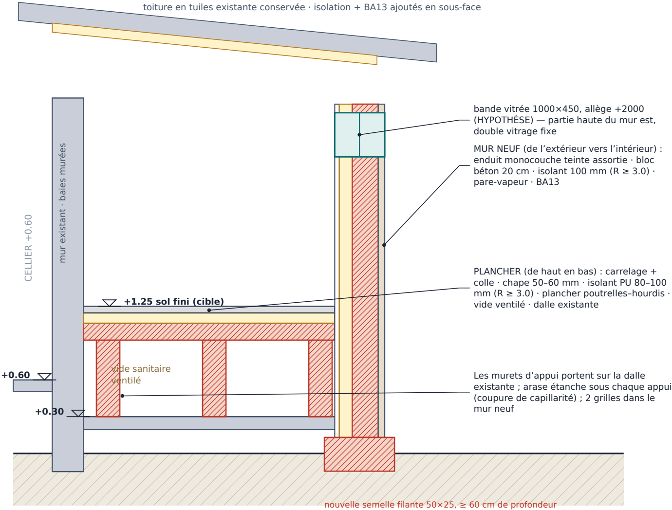
COUPE A-A · ≈ 1:25 @ A3 · vue vers le nord
