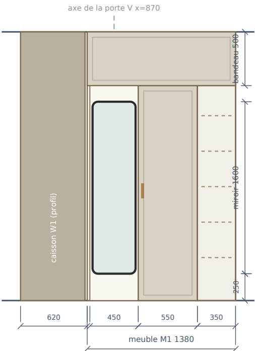
ÉLÉVATION M1 · ≈ 1:35 @ A3
