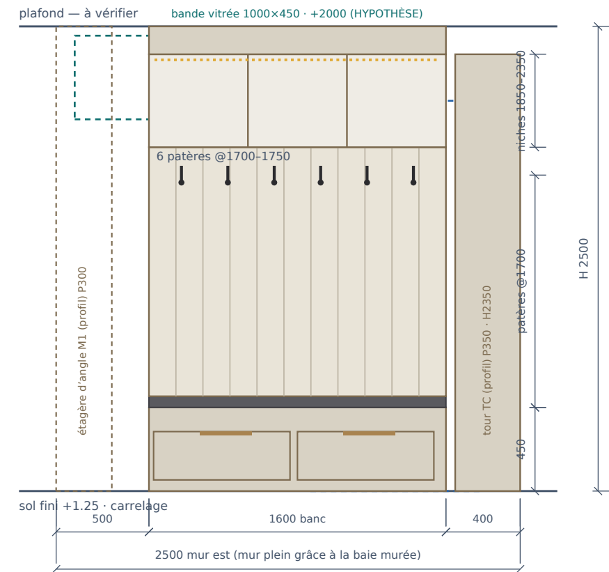
ÉLÉVATION B1 · ≈ 1:28 @ A3 — banc 1600 · 2 tiroirs · 6 patères · 3 niches
