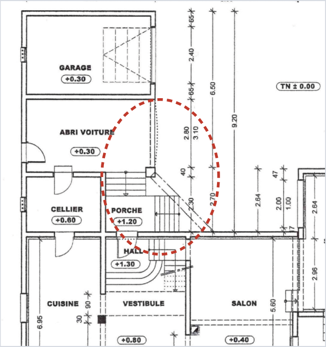
4 · Extrait du plan du permis (2006), RDC — zone du porche
