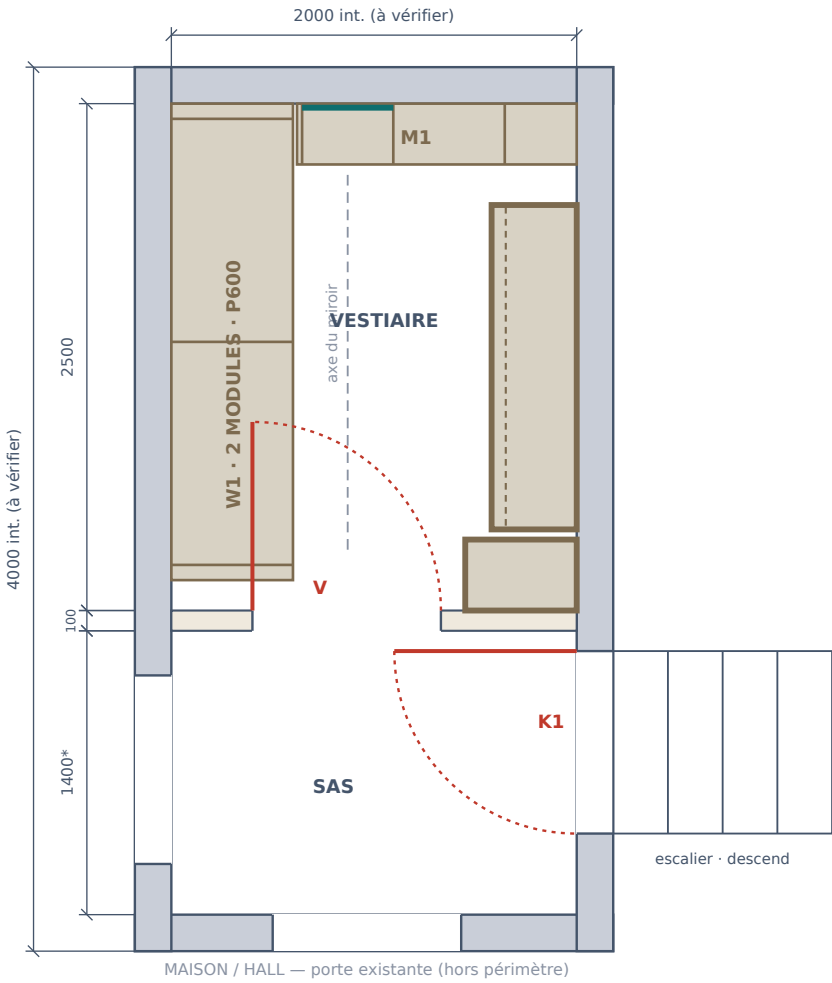
PLAN D'AGENCEMENT (RÉV. B) · ≈ 1:37 @ A3 passage net entre les portes de W1 et le banc B1 ≈ 980 mm · *profondeur du sas : HYPOTHÈSE
