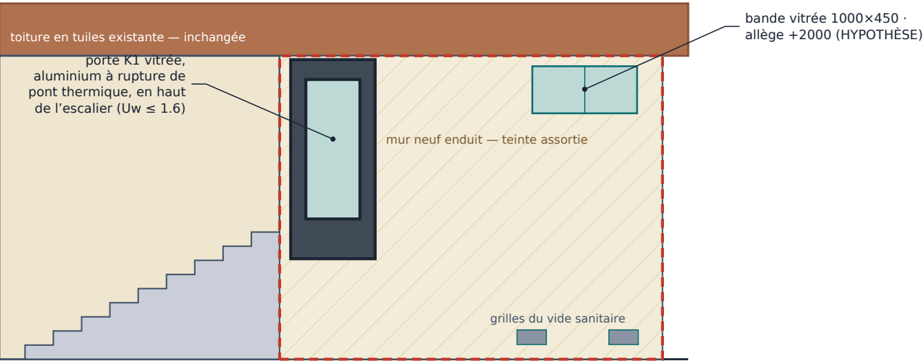
PROJET · façade d’entrée · ≈ 1:60
