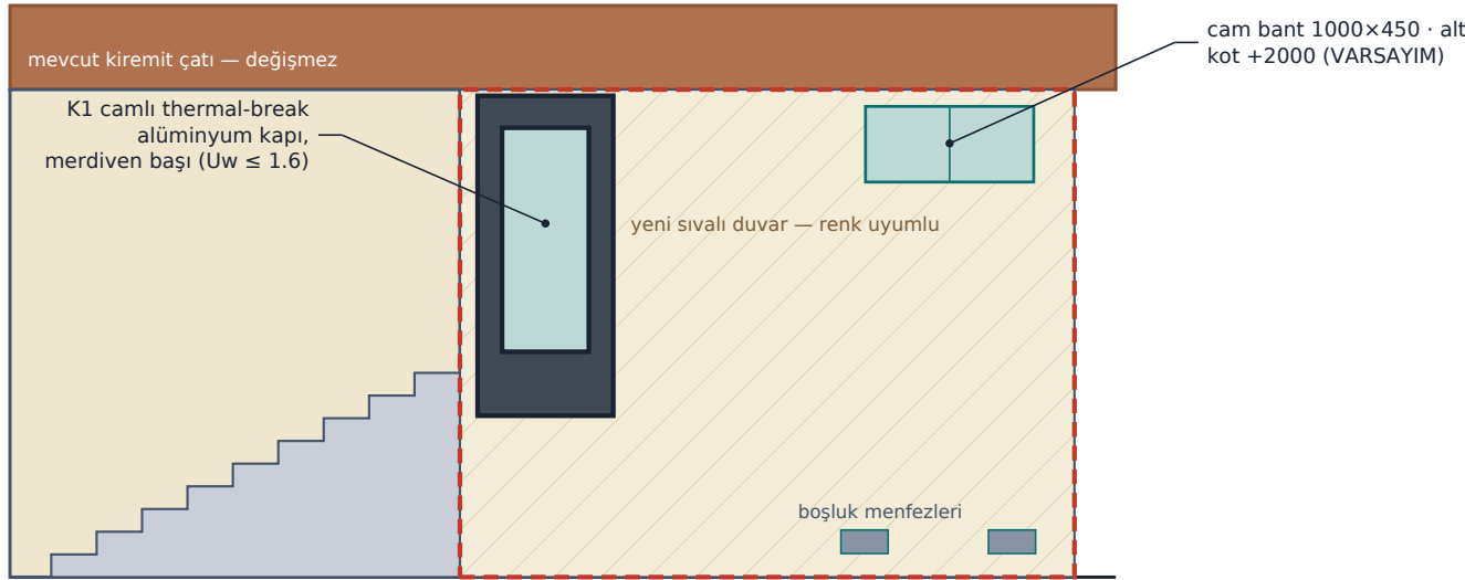
ÖNERİ · giriş cephesi · ≈ 1:60
