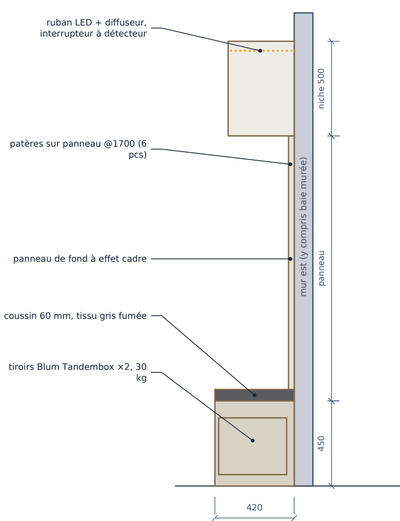
COUPE 1 — MUR BANQUETTE B1 · 1:20
