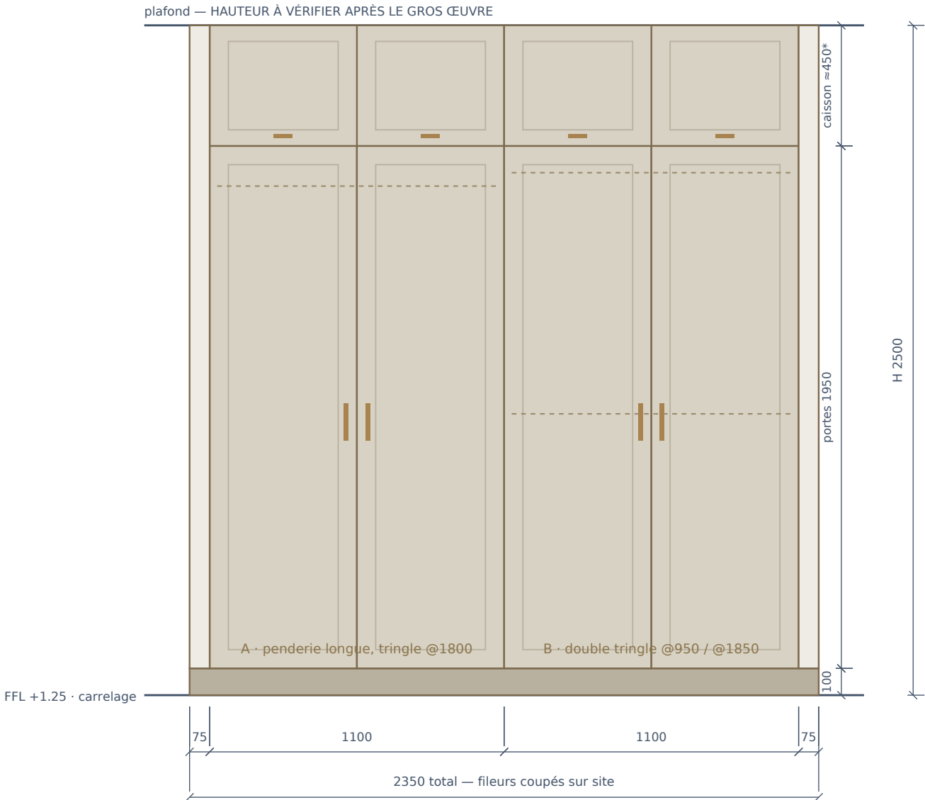
ÉLÉVATION W1 (VUE VERS L'OUEST) · 1:20 — 2 modules à 2 portes de 1100 · portes 1950 + caissons hauts · caissons prof. 600
