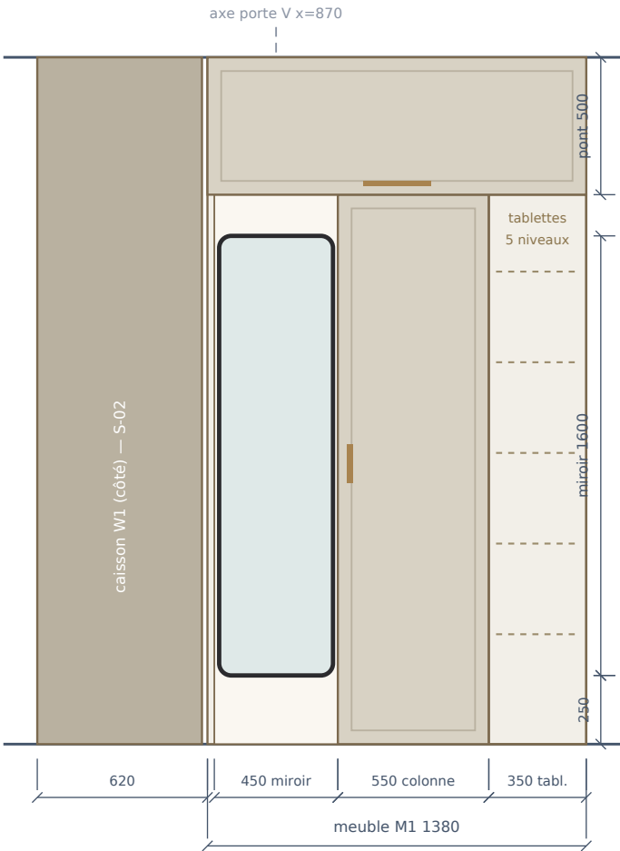
M1 MUR MIROIR — ÉLÉVATION MUR NORD · 1:25
