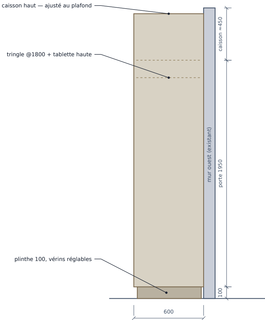
COUPE 2 — PENDERIE HAUTE W1 · 1:20
