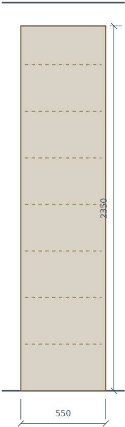
COLONNE CHAUSSURES · 1:25
