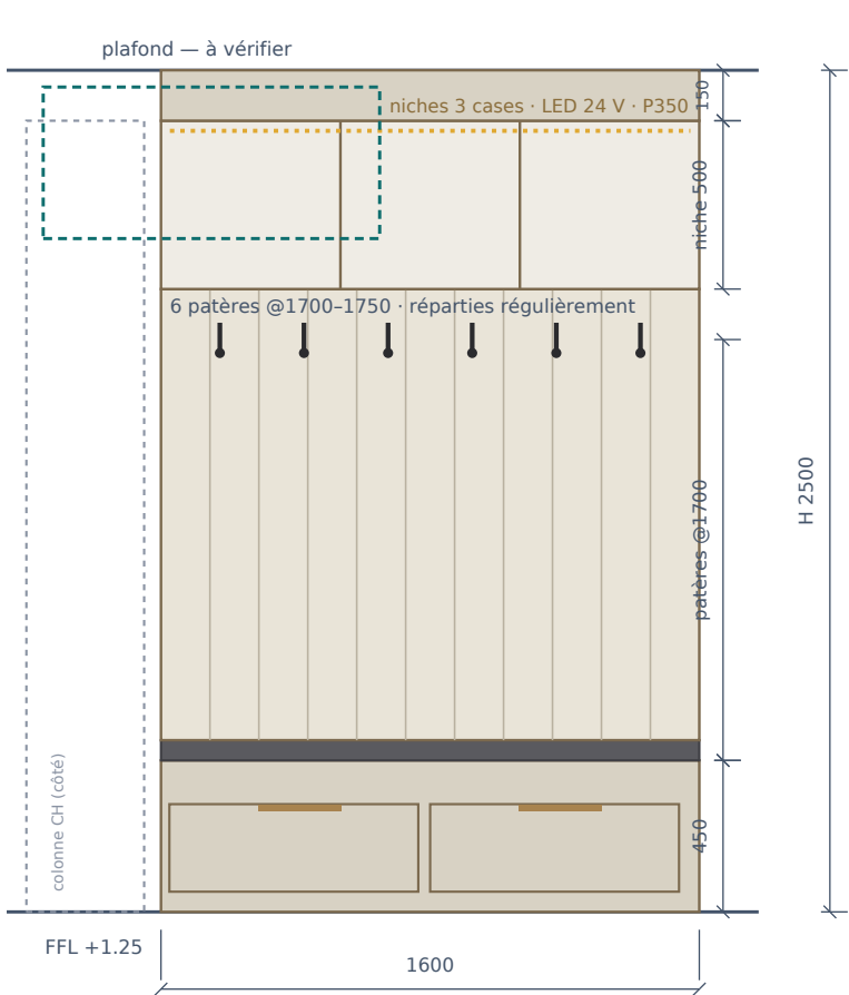
ÉLÉVATION B1 (VUE VERS L'EST) · 1:25
