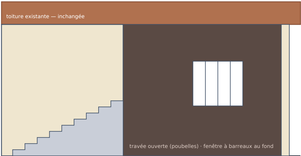
ÉTAT EXISTANT · façade sur voie · ≈ 1:60
