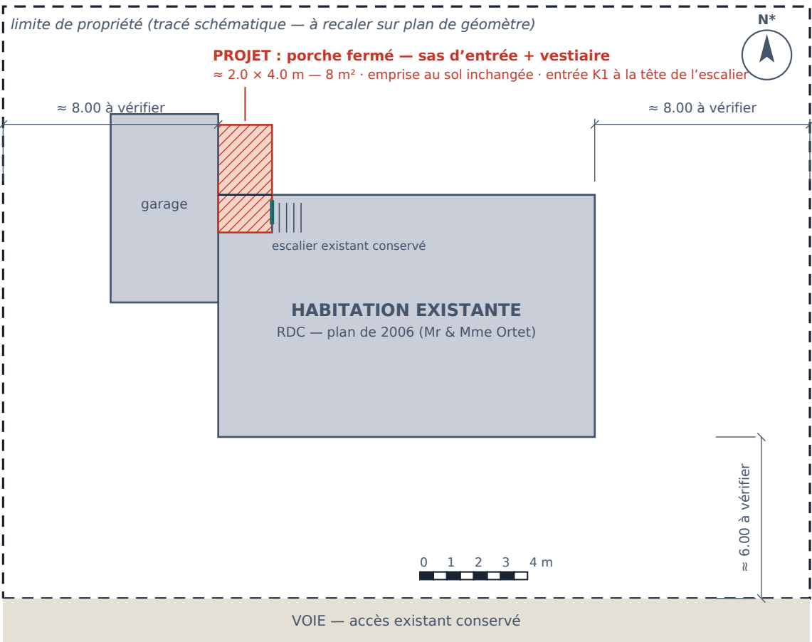
PLAN DE MASSE · ÉCHELLE 1:200 @ A3
