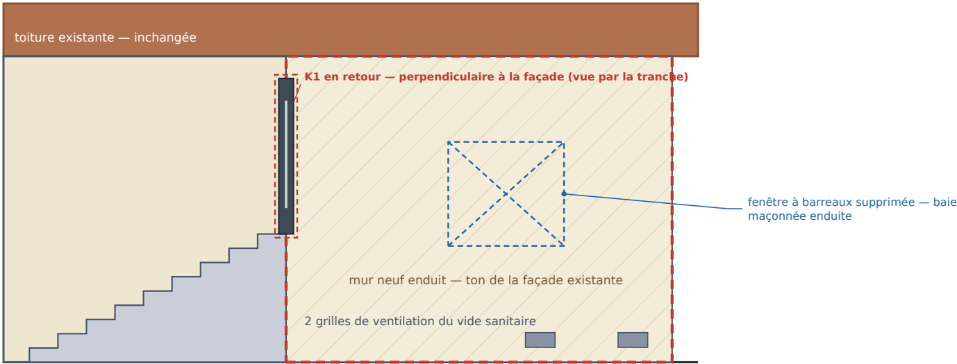
ÉTAT PROJETÉ · façade sur voie · ≈ 1:60
