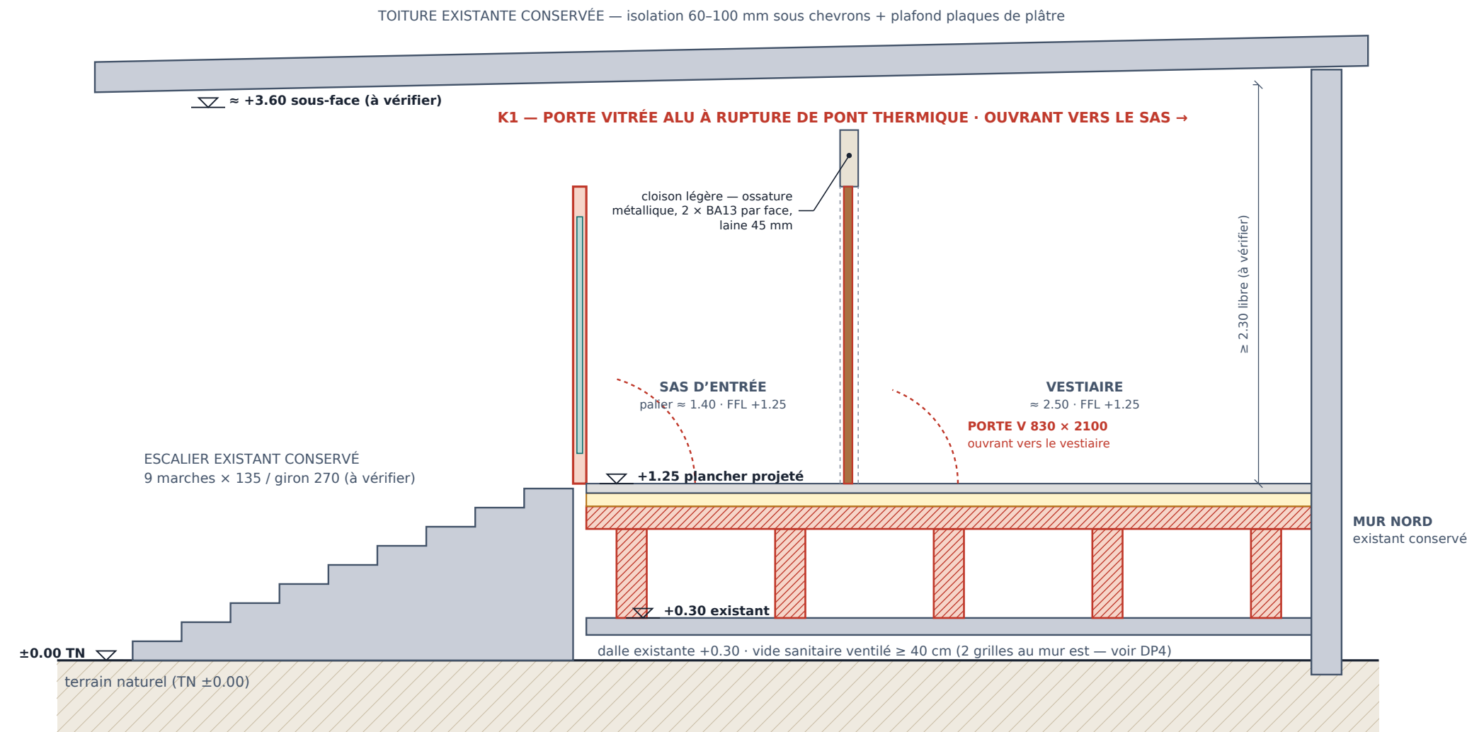
COUPE DÉVELOPPÉE SUR L'ACCÈS (ESCALIER → K1 → SAS → VESTIAIRE) · ÉCHELLE ≈ 1:35 @ A3
