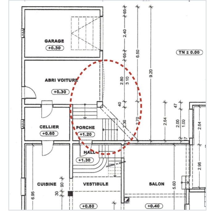
4 · RDC (zemin kat) ruhsat planı paftası (2006) — sundurma bölgesi
