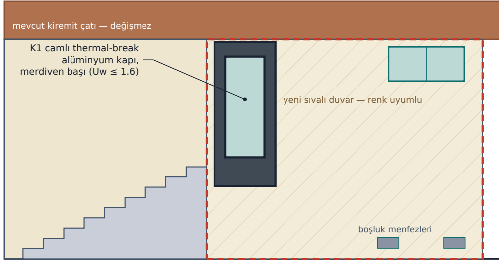
ÖNERİ · giriş cephesi · ≈ 1:60
