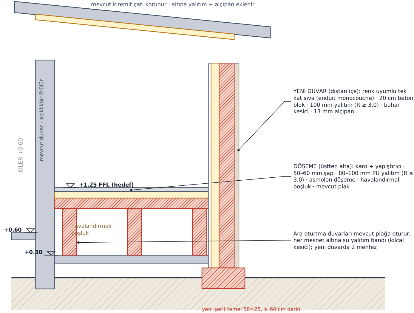
A-A KESİTİ · \approx 1:25 @ A3 · kuzeye bakış
