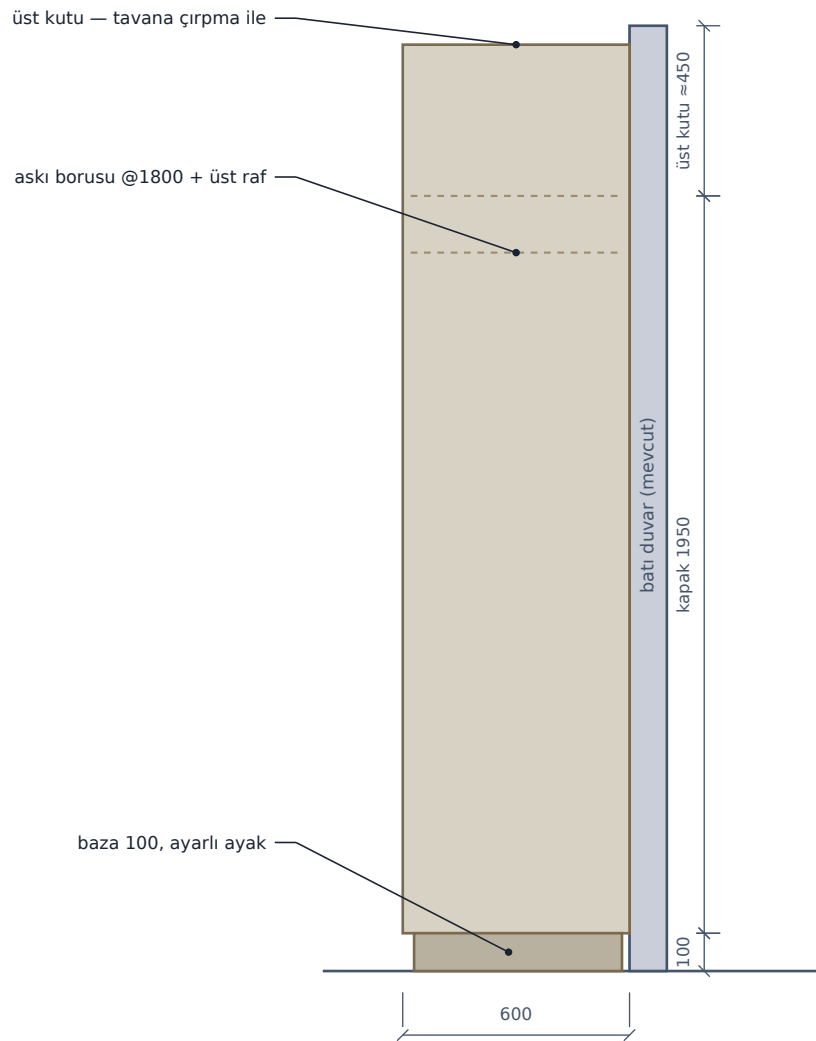
KESİT 2 — BOY DOLAP W1 · 1:20
