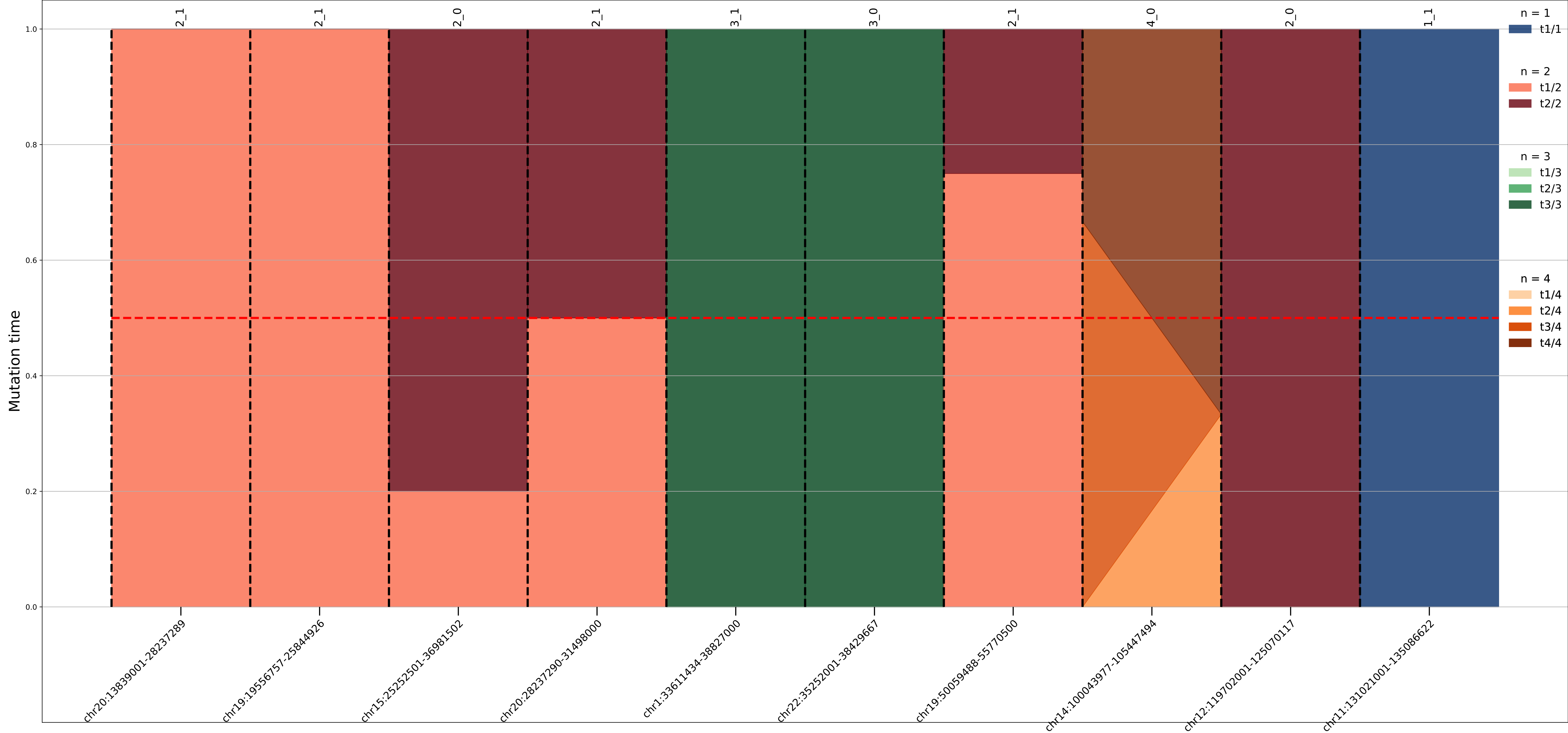
Patient26
