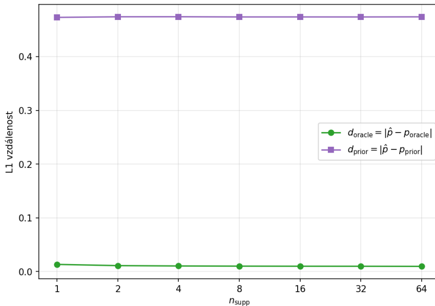
Obrázek 4.13: Vzdálenost predikce PFN od oracly (zelená, p_{\text{oracle}} ) a od uniformní prior masky (fialová, p_{\text{prior}} ), tedy konstantní podíl popředí) jako funkce velikosti kontextu pro náročnou úlohu. Predikce je po celou dobu blízko oracly a daleko od prioru, ke kolapsu nedochází ani při jediném support páru .
