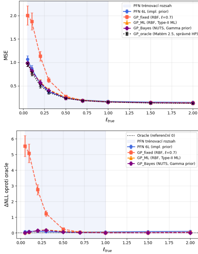
Obrázek 3.20: Vliv síly misspecifikace ( n = 40 ). Nahoře: MSE jako funkce \ell_{\text{true}} . Dole: \Delta\text{NLL} vůči oracle . Modrý pás značí trénovací rozsah PFN \ell \in [0, 0,5, 1, 0] . GP_fixed (oranžová) pro krátké korelační délky selhává v obou metrikách, ostatní metody se s rostoucím \ell_{\text{true}} sbíhají k oracle . PFN zůstává blízko oracle v celém rozsahu včetně hodnot mimo svůj trénovací rozsah.
