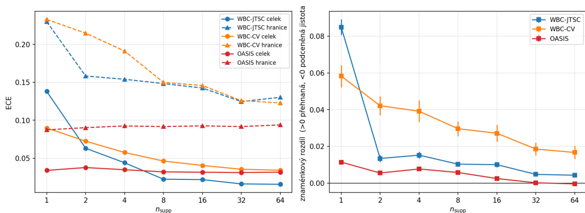
Obrázek 4.6: Vlevo očekávaná kalibrační chyba (ECE) zvlášť pro celý obrázek a pro hraniční pásmo, vpravo znaménkový rozdíl mezi jistotou a správností (kladný znamená přehnanou jistotu). Kalibrační chyba je na hranici řádově vyšší než uvnitř a klesá s kontextem pomaleji.
