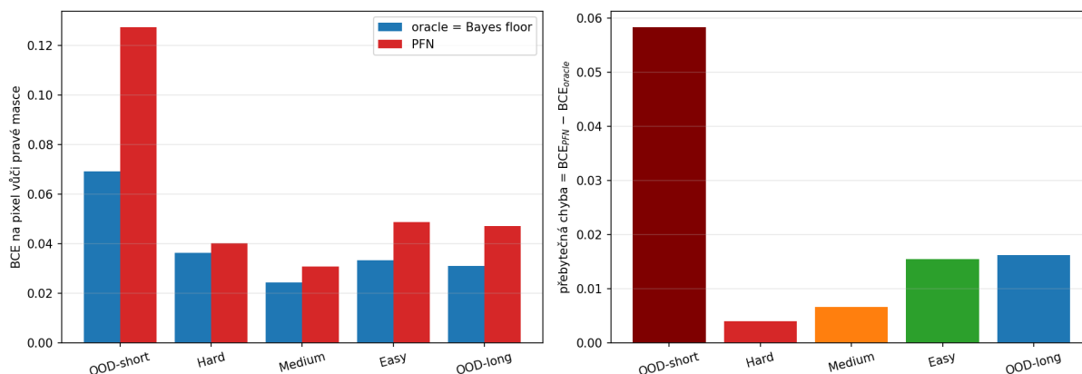
Obrázek 4.12: Vlevo chyba PFN a Bayes floor (chyba samotného oraclu ) pro jednotlivé režimy, měřená binární křížovou entropií (BCE) na pixel. Vpravo jejich rozdíl BCE_{\text{PFN}} - BCE_{\text{oracle}} , tedy přebytečná chyba PFN nad optimem. Uvnitř trénovacího rozsahu je malá, prudce roste jen u členitějších polí mimo rozsah (OOD-short).
