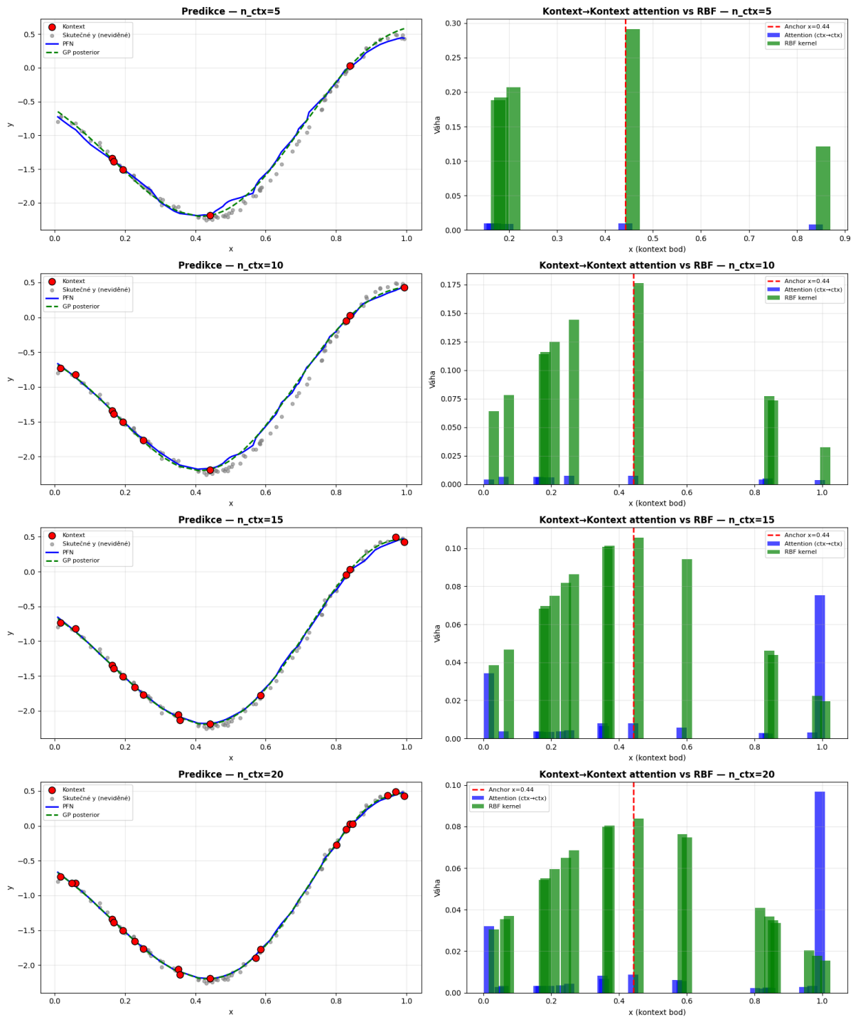
Obrázek 3.10: Náhodný model: predikce (levý sloupec) a attention vs RBF (pravý sloupec) pro n \in \{5, 10, 15, 20\} . Červené body: kontext; šedé: skutečné neviděné hodnoty; modrá: PFN; zelená přerušovaná: GP se správným \ell .
