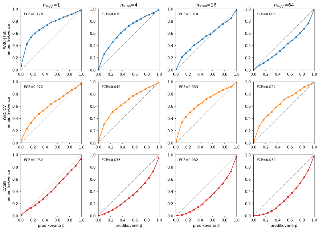
Obrázek 4.5: Reliability diagramy pro tři domény (řádky) a vybrané velikosti support setu (sloupce). Křivka nad úhlopříčkou znamená podhodnocenou jistotu, pod úhlopříčkou přehnanou. Krvinky (WBC) leží nad úhlopříčkou, mozek (OASIS) pod ní.
