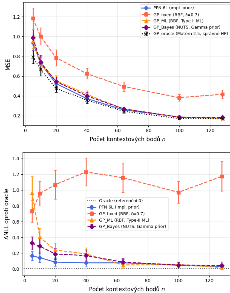
Tabulka 3.15: MSE vůči skutečným hodnotám jako funkce velikosti kontextu n při misspecifikaci kernelu ( \ell_{\text{true}} = 0,3 , průměr přes 150 instancí). PFN je pro n \in \{10, 20, 40\} nejlepší ze všech misspecifikovaných metod, pro velká n je s GP_ML a GP_Bayes prakticky shodné.
