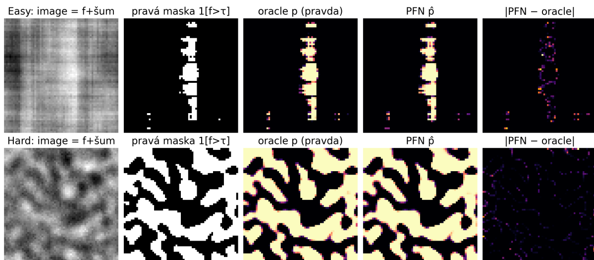
Obrázek 4.7: Ukázka predikcí pro snadnou (nahore) a náročnou (dole) úlohu. Zleva vstupní obrázek, pravá maska, oracle (pravý posterior), predikce PFN a jejich absolutní rozdíl. Mapy PFN a oracle u téměř splývají, rozdíl je soustředěn na hranici mezi popředím a pozadím, tedy na obrysu segmentované oblasti.
