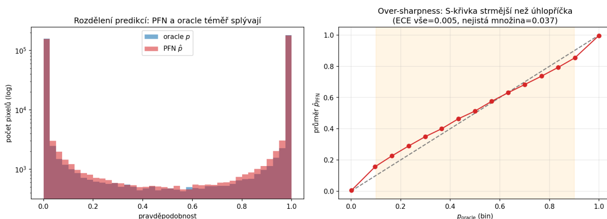
Obrázek 4.9: Vlevo rozdělení predikovaných pravděpodobností PFN a oracul přes všechny pixely, obě křivky se téměř překrývají. Vpravo srovnání průměrné predikce PFN s oraclem po intervalech, mírné vybočení od úhlopříčky odpovídá přehnané ostrosti na hranicích.
