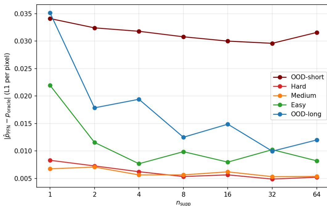
Obrázek 4.8: Průměrná vzdálenost predikce PFN od oracle u jako funkce velikosti kontextu pro pět režimů náročnosti. Uvnitř trénovacího rozsahu (Hard, Medium, Easy) je vzdálenost malá a na velikosti kontextu skoro nezávisí. Mimo rozsah (OOD-short, OOD-long) je větší, členitější pole (OOD-short) model nedožene ani s velkým kontextem.
