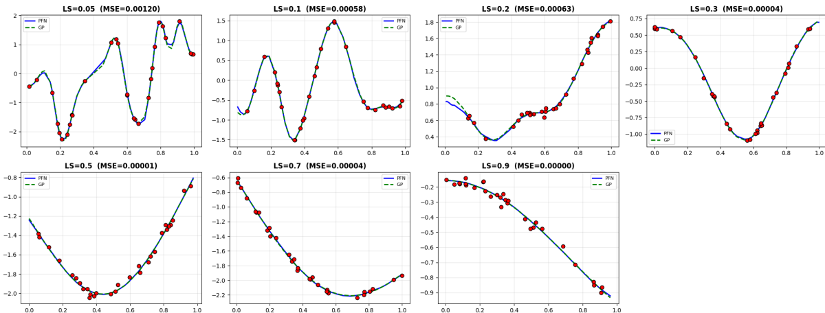
(b) Vizualizace predikcí pro různé \ell . Pro malé \ell (rychlé oscilace) PFN ztlačně přehlazuje, pro velké \ell sleduje GP posterior téměř dokonale.
