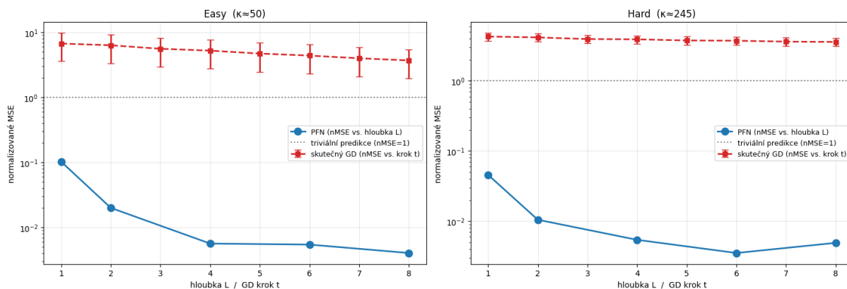
Obrázek 3.17: PFN versus skutečný gradientní sestup, obojí v predikčním prostoru, pro Easy (vlevo) a Hard (vpravo). Modrá: normalizované MSE PFN proti hloubce L . Červená: normalizované MSE gradientního sestupu proti počtu kroků t (stejně osy). Tečkovaná čára značí triviální predikci konstantním průměrem (nMSE = 1). PFN je hluboko pod triviální úrovní už při jedné vrstvě, zatímco skutečný gradientní sestup zůstává nad triviální predikcí i po osmi krocích.
