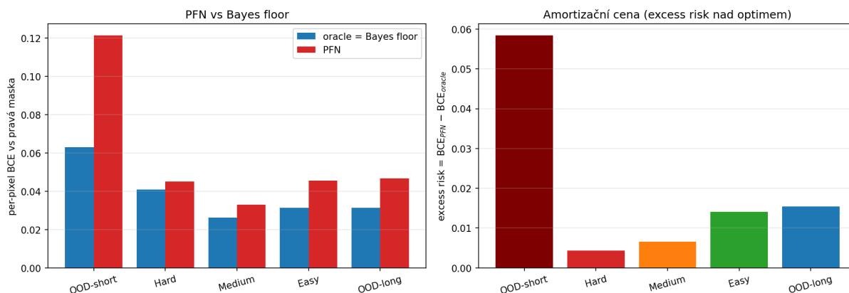
Obrázek 4.12: Vlevo chyba PFN a Bayes floor (chyba samotného oraculu ) pro jednotlivé režimy, měřena binární křížovou entropií (BCE) na pixel. Vpravo jejich rozdíl BCE_{PFN} - BCE_{oracle} , v grafu označený excess risk , tedy přebytečná chyba PFN nad optimem. Uvnitř trénovacího rozsahu je malá, prudce roste jen u členitějších polí mimo rozsah (OOD-short).
