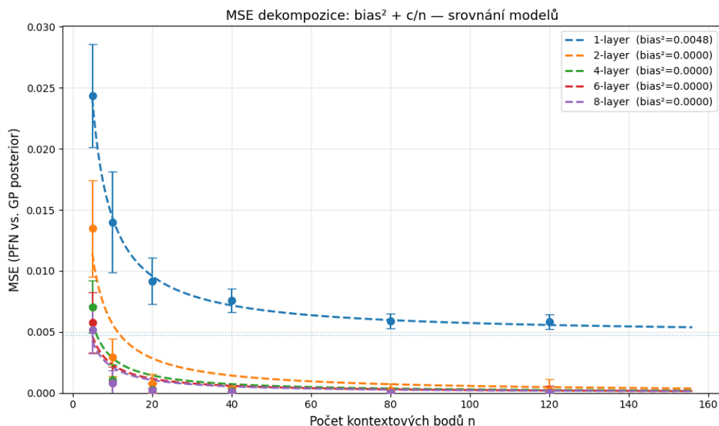
Obrázek 3.15: Rozklad MSE = bias^2 + c/n pro všech pět modelů. Body jsou naměřené MSE (chybové úsečky \pm 1 \text{ std} ), přerušované křivky proložení. Jednovrstvý model (modrá) se s rostoucím n vyrovnává na nenulové asymptotě bias^2 = 0,0048 (tečkovaná čára), zatímco hlubší modely klesají prakticky k nule. Rozdíly mezi 4, 6 a 8 vrstvami jsou už zanedbatelné.
