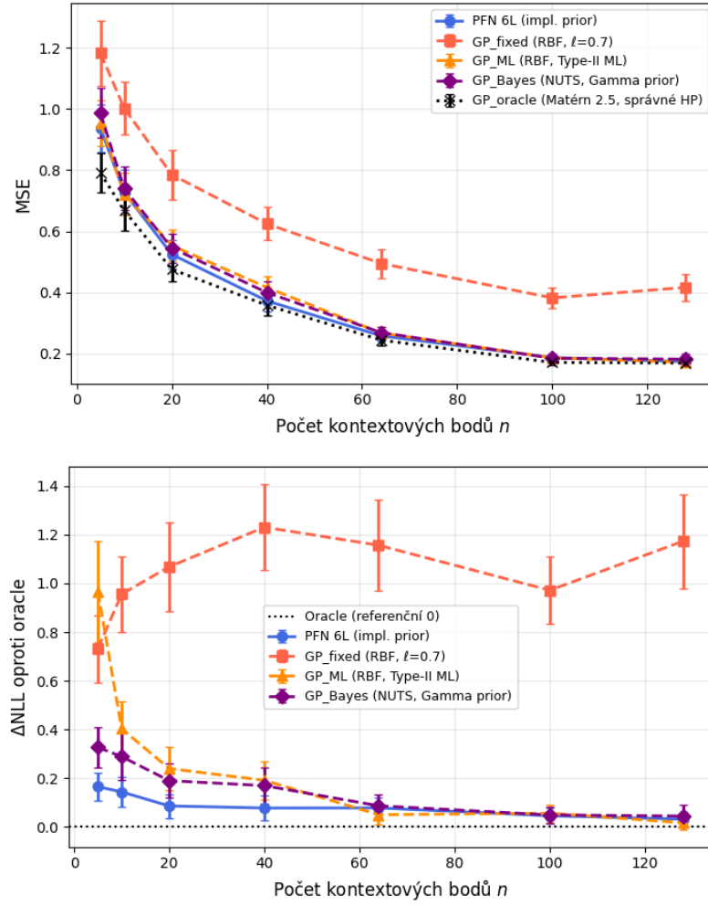
Obrázek 3.19: Vliv velikosti kontextu při misspecifikaci kernelu (data z Matérn 2,5, \ell_{\text{true}} = 0,3 ). Nahoře: MSE jako funkce n , černá tečkovaná čára je GP_{\text{oracle}} . Dole: \Delta NLL vůči oracle , tečkovaná čára značí nulu ( oracle ). Chybové úsečky \pm 1 směrodatná chyba. PFN (modrá) se v MSE drží těsně u oracle a v \Delta NLL je pro malé a střední kontexty ze všech metod nejnižší.
