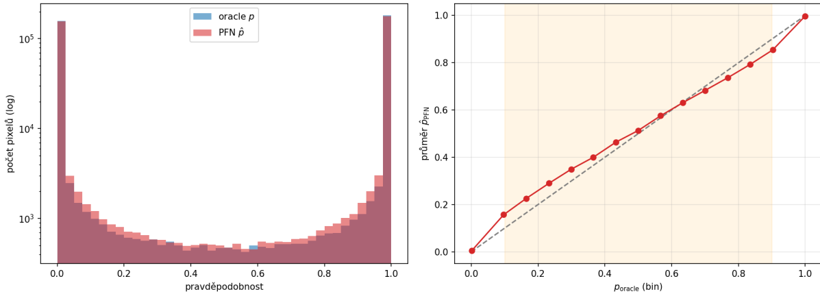
Obrázek 4.9: Vlevo rozdělení predikovaných pravděpodobností PFN a oraclu přes všechny pixely, obě křivky se téměř překrývají. Vpravo srovnání průměrné predikce PFN s oraclem po intervalech, mírné vybočení od úhlopříčky odpovídá přehnané ostrosti na hranicích.
