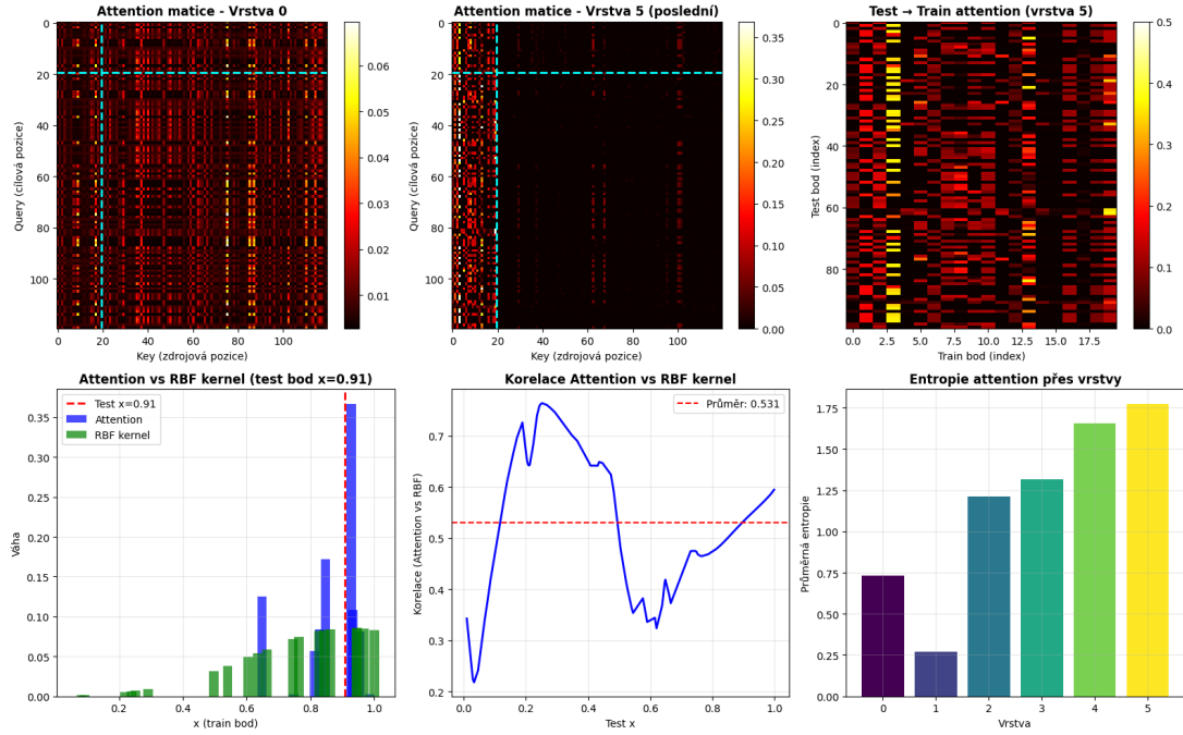
Obrázek 3.2: Detailní rozbor attention fixního modelu (průměr přes 8 hlav). Nahoře: attention matice vrstvy 0 a poslední vrstvy 5 a výřez bloku Test → Train poslední vrstvy. Dole vlevo: attention váhy pro vybraný testovací bod v porovnání s normalizovanými RBF vahami, attention je výrazně ostřejší, koncentruje téměř veškerou váhu na nejbližší bod, zatímco RBF distribuuje váhu plynule. Dole uprostřed: korelace attention s RBF jako funkce polohy testovacího bodu. Dole vpravo: průměrná entropie attention vah po vrstvách.
