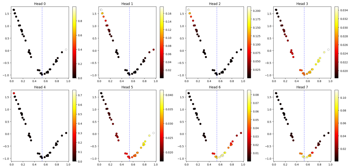
Obrázek 3.13: Iso-weight rozklad jednovrstvého modelu na 8 hlav. Pro pevný testovací bod x^* = 0,54 (modrá přerušovaná čára) je každý kontextový bod vynesen do roviny (X_j, Y_j) a obarven attention vahou dané hlavy (světlejší = vyšší). Kernelové porovnání by koncentrovalo váhu kolem x^* nezávisle na Y_j . Místo toho různé hlavy míří do různých rohů roviny (X, Y) , tedy na různé hodnoty Y_j , což je přímý vizuální doklad, že attention závisí i na labelu . Hlavy 0, 4, 6 navíc degenerují na jediný bod ( attention sink ).
