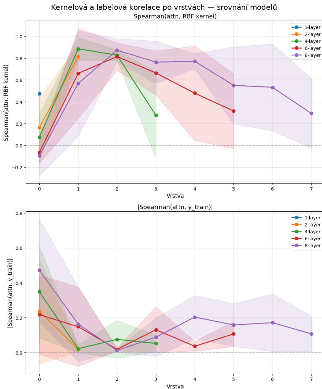
Obrázek 3.11: Srovnání všech pěti modelů. Nahoře: Spearmanova korelace attention vah s RBF kernelem jako funkce indexu vrstvy. Dole: absolutní hodnota korelace attention vah s labels Y_j . Barevné pásy značí \pm 1 směrodatnou odchylku přes hlavy. Vzor je u všech modelů stejný: vrstva 0 má nejvyšší labelovou a nejnižší kernelovou korelaci, střední vrstvy se chovají kernel-like (vysoká kernelová , nízká labelová korelace) a v poslední vrstvě kernelová korelace opět klesá.
