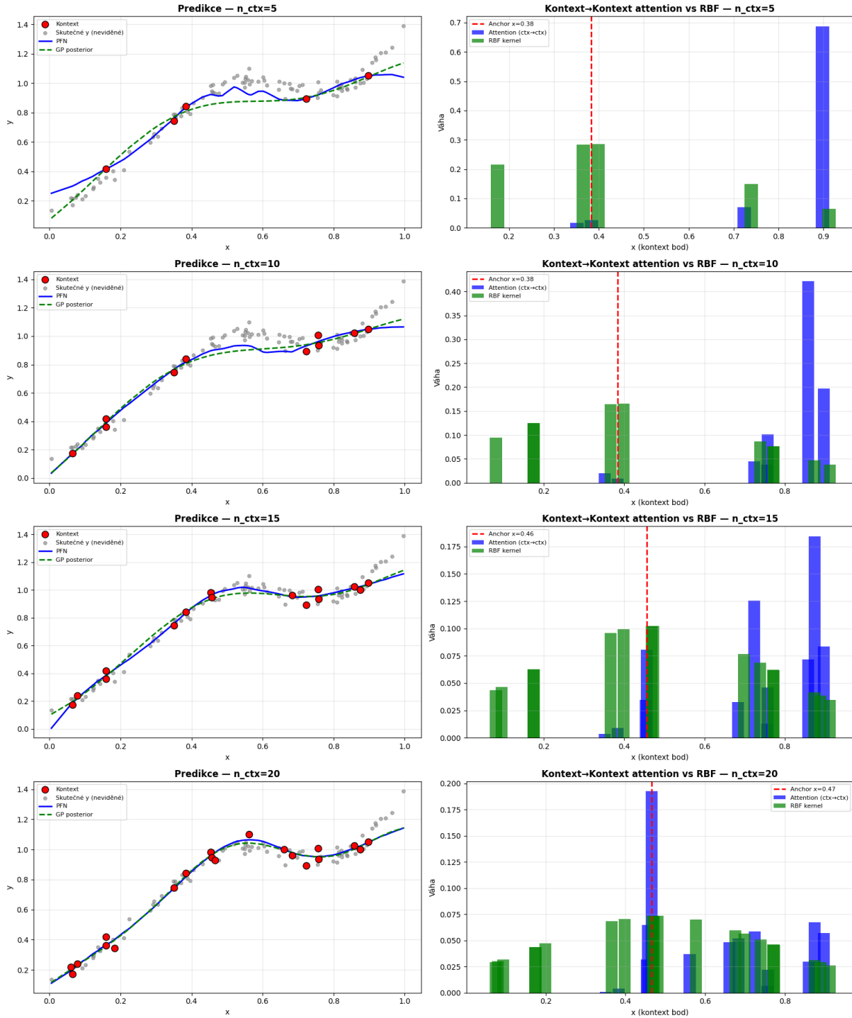
Obrázek 3.4: Vizualizace predikcí (levý sloupec) a attention vs RBF (pravý sloupec) pro n \in \{5, 10, 15, 20\} . Červené body: kontextová data dostupná modelu; šedé body: skutečné neviděné hodnoty; modrá: PFN; zelená přerušovaná: GP posterior se správným \ell . Všechny řádky vychází ze stejné GP realizace, liší se pouze velikostí kontextu. Od n = 15 obě křivky téměř splývají.
