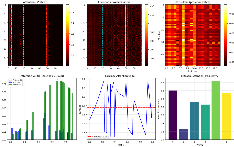
Obrázek 3.7: Detailní rozbor attention náhodného modelu (průměr přes 8 hlav). Nahoře: attention matice vrstvy 0 a poslední vrstvy a výřez bloku Test → Train . Dole vlevo: attention váhy (modrá) pro vybraný testovací bod v porovnání s normalizovanými RBF vahami (zelená). Dole uprostřed: korelace attention s RBF jako funkce polohy testovacího bodu. Dole vpravo: průměrná entropie attention vah po vrstvách. Stejně jako u fixního modelu je attention výrazně ostřejší a s RBF nekoreluje (korelace 0,316 \pm 0,311 ).
