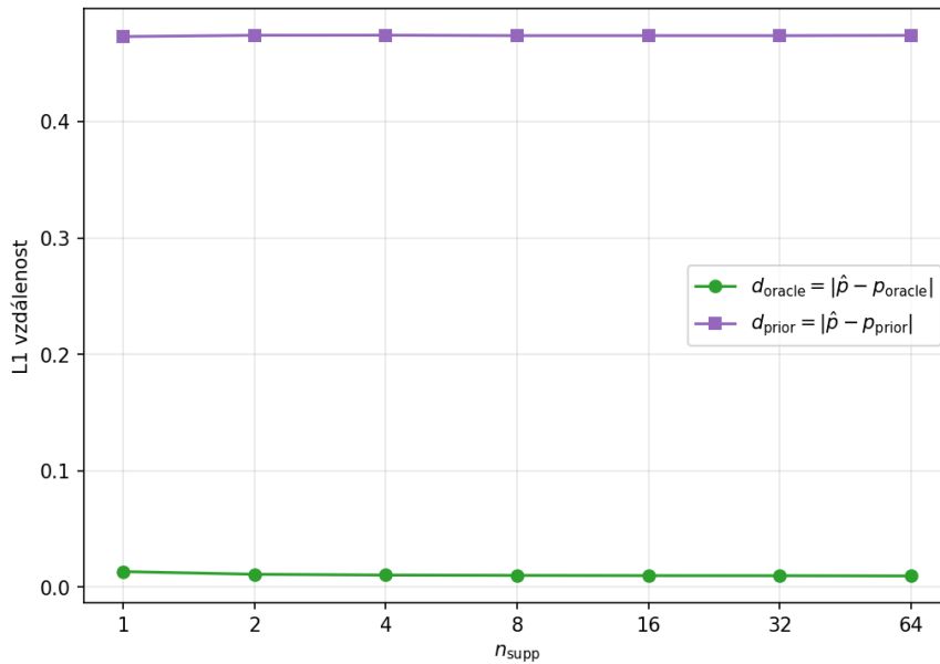
Obrázek 4.13: Vzdálenost predikce PFN od oraclu (zelená, p_{\text{oracle}} ) a od uniformní prior masky (fialová, p_{\text{prior}} , tedy konstantní podíl popředí) jako funkce velikosti kontextu pro náročnou úlohu. Predikce je po celou dobu blízko oraclu a daleko od prioru, ke kolapsu nedochází ani při jediném support páru .
