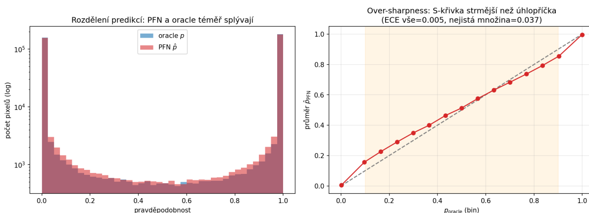
Obrázek 4.9: Vlevo rozdělení predikovaných pravděpodobností PFN a oraclo přes všechny pixely, obě křivky se téměř překrývají. Vpravo srovnání průměrné predikce PFN s oraclem po intervalech, mírné vybočení od úhlopříčky odpovídá přehnané ostrosti na hranicích.
