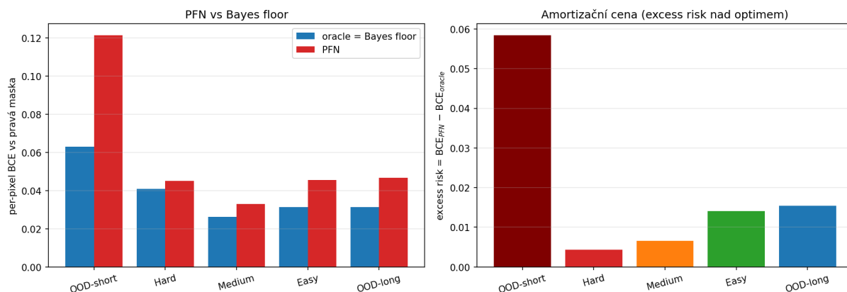
Obrázek 4.12: Vlevo chyba PFN a Bayes floor (chyba samotného oraculu ) pro jednotlivé režimy, měřená binární křížovou entropií (BCE) na pixel. Vpravo jejich rozdíl BCE_{PFN} - BCE_{Oracle} , v grafu označený excess risk , tedy přebytková chyba PFN nad optimem. Uvnitř trénovacího rozsahu je malá, prudce roste jen u členitějších polí mimo rozsah (OOD-short).
