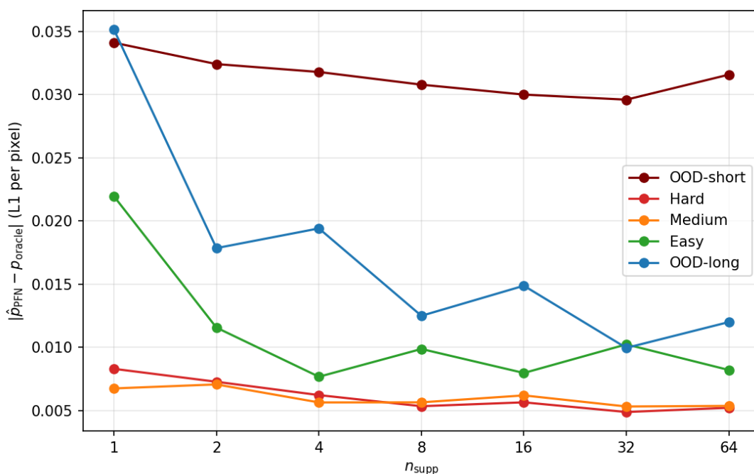
Obrázek 4.8: Průměrná vzdálenost predikce PFN od oraclu jako funkce velikosti kontextu pro pět režimů náročnosti. Uvnitř trénovacího rozsahu (Hard, Medium, Easy) je vzdálenost malá a na velikosti kontextu skoro nezávisí. Mimo rozsah (OOD-short, OOD-long) je větší, členitější pole (OOD-short) model nedožene ani s velkým kontextem.
