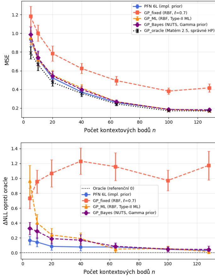
Obrázek 3.19: Vliv velikosti kontextu při misspecifikaci kernelu (data z Matérn 2,5, \ell_{\text{true}} = 0,3 ). Nahoře: MSE jako funkce n , černá tečkovaná čára je GP_{\text{oracle}} . Dole: \Delta\text{NLL} vůči oracle , tečkovaná čára značí nulu ( oracle ). Chybové úsečky \pm 1 směrodatná chyba. PFN (modrá) se v MSE drží těsně u oracle a v \Delta\text{NLL} je pro malé a střední kontexty ze všech metod nejnižší.
