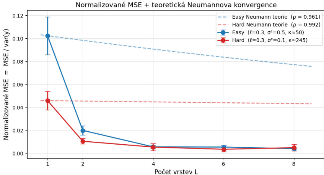
Obrázek 3.17: Normalizované MSE jako funkce hloubky L pro oba režimy (plné čáry, chybové úsečky \pm 1 směrodatná chyba) proti teoretické křivce \rho^L , tedy nejpomalejšímu poklesu, který teorie gradientnímu sestupu v nejhorším případě předpovídá (přerušované čáry). Chyba prudce klesá s hloubkou, u Easy z 0,10 na 0,004, u Hard z 0,046 na 0,005, a hlavní zisk se odehrává mezi jednou a čtyřmi vrstvami. Empirický pokles je ovšem mnohem rychlejší než teoretická křivka, už 2–4 vrstvy dosáhnou přesnosti, kterou by Neumannova řada nedala ani po desítkách kroků.
