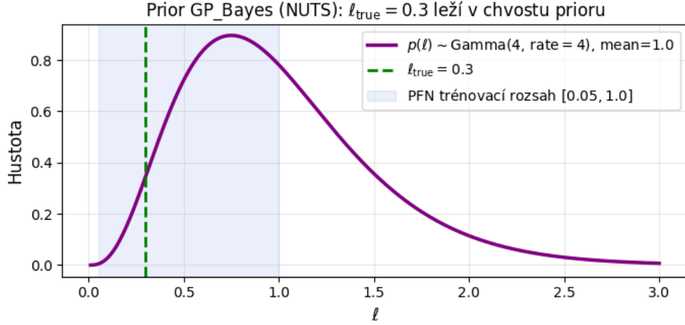
Obrázek 3.19: Prior p(\ell) \sim \text{Gamma}(4, 4) metody GP_Bayes (fialová) se střední hodnotou u \ell = 1,0 . Zelená přerušovaná čára značí pravou hodnotu \ell_{\text{true}} = 0,3 , která leží v chvostu prioru. Modrý pás vyznačuje trénovací rozsah PFN \ell \in [0,05, 1,0] , pravá hodnota leží uvnitř něj.
