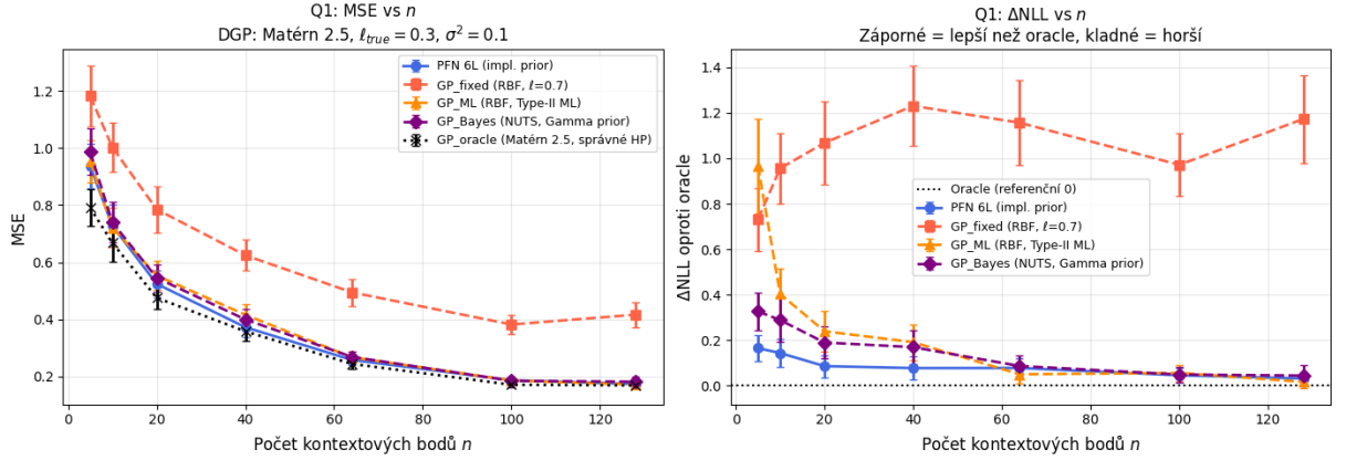
Obrázek 3.20: Vliv velikosti kontextu při misspecifikaci kernelu (data z Matérn 2,5, \ell_{\text{true}} = 0,3 ). Vlevo: MSE jako funkce n , černá tečkovaná čára je GP_{\text{oracle}} . Vpravo: \Delta\text{NLL} vůči oracle , tečkovaná čára značí nulu ( oracle ). Chybové úsečky \pm 1 směrodatná chyba. PFN (modrá) se v MSE drží těsně u oracle a v \Delta\text{NLL} je pro malé a střední kontexty ze všech metod nejnižší.
