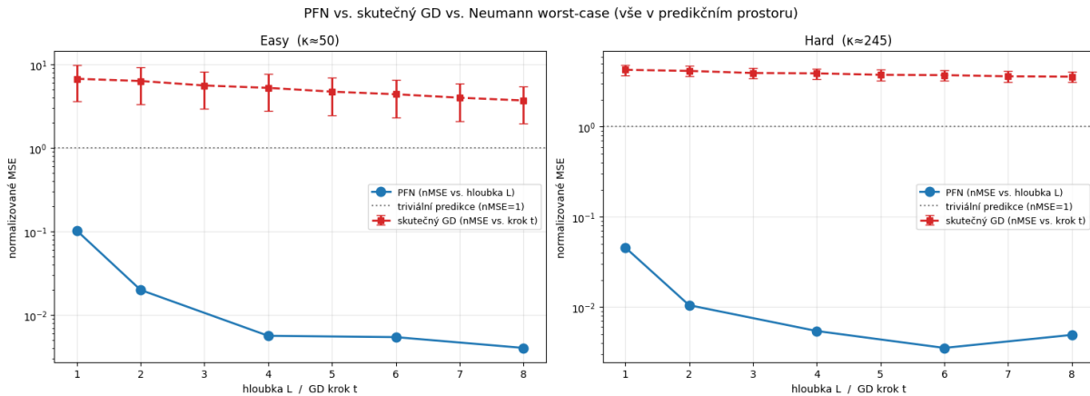
Obrázek 3.18: PFN versus skutečný gradientní sestup, obojí v predikčním prostoru, pro Easy (vlevo) a Hard (vpravo). Modrá: normalizované MSE PFN proti hloubce L . Červená: normalizované MSE gradientního sestupu proti počtu kroků t (stejně osy). Tečkovaná čára značí triviální predikci konstantním průměrem ( \text{nMSE} = 1 ). PFN je hluboko pod triviální úrovní už při jedné vrstvě, zatímco skutečný gradientní sestup zůstává nad triviální predikcí i po osmi krocích.
