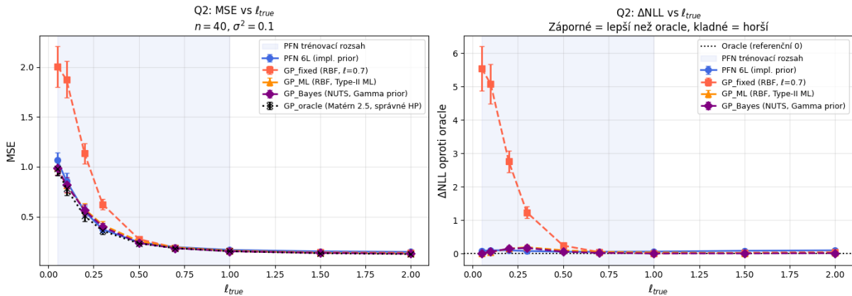
Obrázek 3.21: Vliv síly misspecifikace ( n = 40 ). Vlevo: MSE jako funkce \ell_{\text{true}} . Vpravo: \Delta\text{NLL} vůči oracle . Modrý pás značí trénovací rozsah PFN \ell \in [0,05, 1,0] . GP_fixed (oranžová) pro krátké korelační délky selhává v obou metrikách, ostatní metody se s rostoucím \ell_{\text{true}} sbíhají k oracle . PFN zůstává blízko oracle v celém rozsahu včetně hodnot mimo svůj trénovací rozsah.
