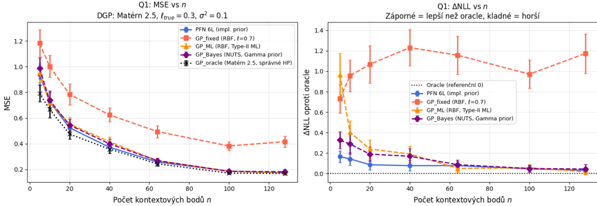
Obrázek 3.19: Vliv velikosti kontextu při misspecifikaci kernelu (data z Matérn 2,5, \ell_{\text{true}} = 0,3 ). Vlevo: MSE jako funkce n , černá tečkovaná čára je GP\_oracle . Vpravo: \Delta\text{NLL} vůči oracle , tečkovaná čára značí nulu ( oracle ). Chybové úsečky \pm 1 směrodatná chyba. PFN (modrá) se v MSE drží těsně u oracle a v \Delta\text{NLL} je pro malé a střední kontexty ze všech metod nejnižší.
