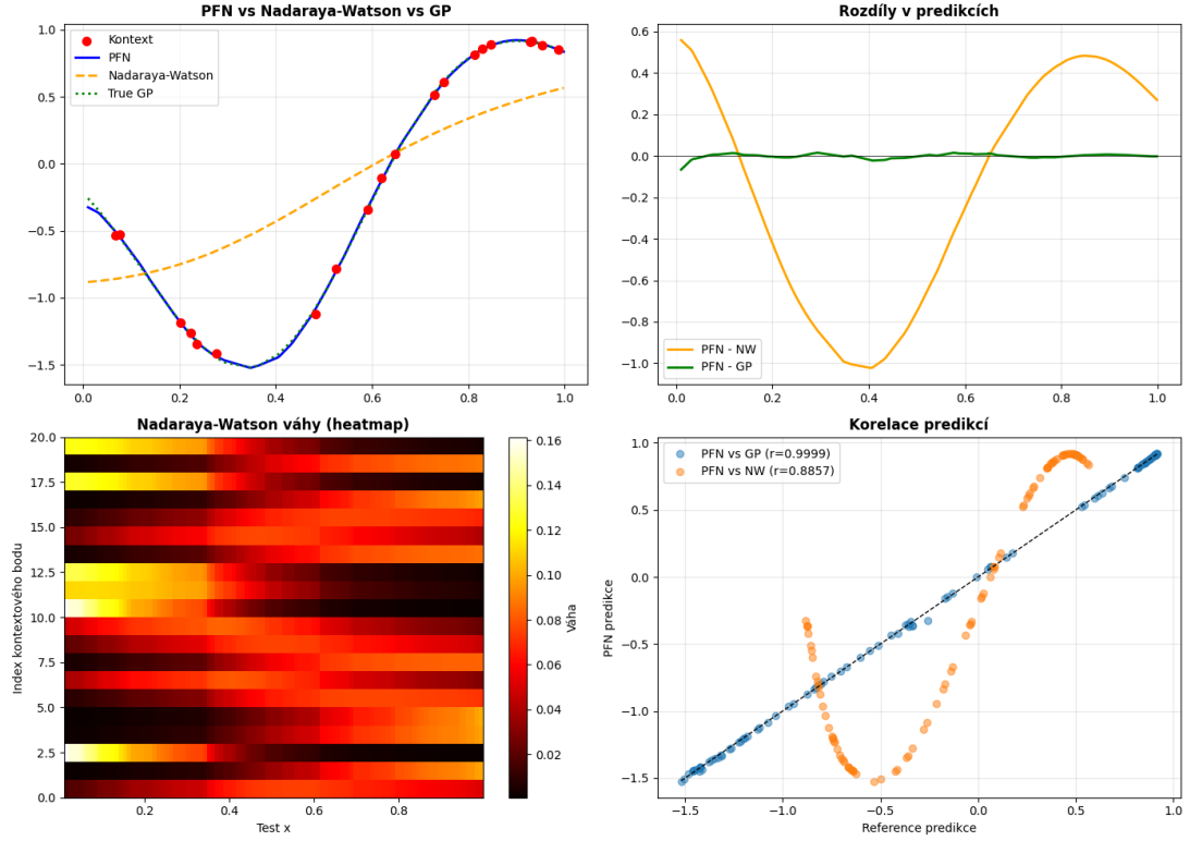
Obrázek 3.3: Srovnání predikcí PFN, Nadaraya-Watsonova estimátoru a analytického GP posterioru ( n_{\text{ctx}} = 20 ). NW systematicky přehlazuje, zatímco PFN sleduje GP posterior těsně, přesné hodnoty MSE shrnuje tabulka 3.1.
