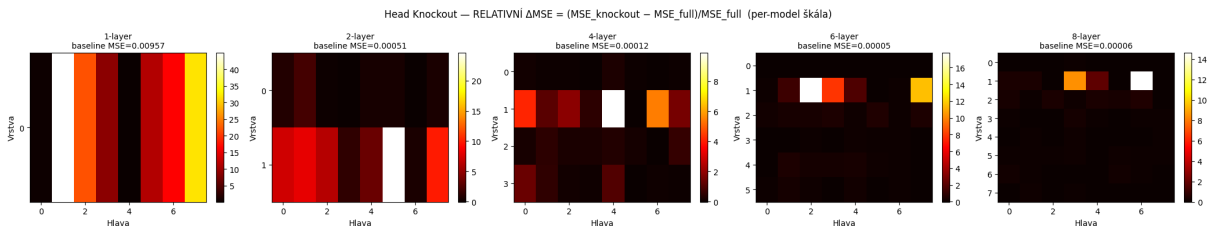
Obrázek 3.14: Head-knockout pro všech pět modelů. Každá teplotní mapa zobrazuje relativní zhoršení \text{rel} = (\text{MSE}_{\text{knockout}} - \text{MSE}_{\text{full}}) / \text{MSE}_{\text{full}} (světlejší = důležitější) po vynulování hlavy na dané pozici (vrstva \times hlava). Každý model má vlastní barevnou škálu, jinak by hluboké modely s malou baseline chybou byly celé tmavé. Kauzálně důležité hlavy se koncentrují do raných vrstev (vrstva 0–1) napříč všemi modely. Jednovrstvý model je nejkřehčí (až 44,9× baseline ), ale i hluboké modely nesou odebrání jediné hlavy 10 až 25× vlastní baseline chyby .
