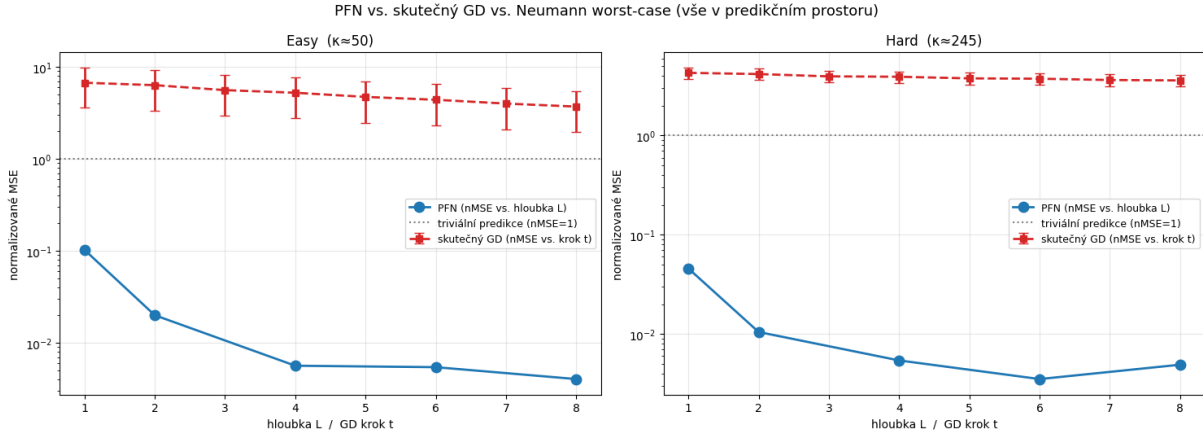
Obrázek 3.17: PFN versus skutečný gradientní sestup, obojí v predikčním prostoru, pro Easy (vlevo) a Hard (vpravo). Modrá: normalizované MSE PFN proti hloubce L . Červená: normalizované MSE gradientního sestupu proti počtu kroků t (stejně osy). Tečkovaná čára značí triviální predikci konstantním průměrem ( \text{nMSE} = 1 ). PFN je hluboko pod triviální úroveň už při jedné vrstvě, zatímco skutečný gradientní sestup zůstává nad triviální predikcí i po osmi krocích.
