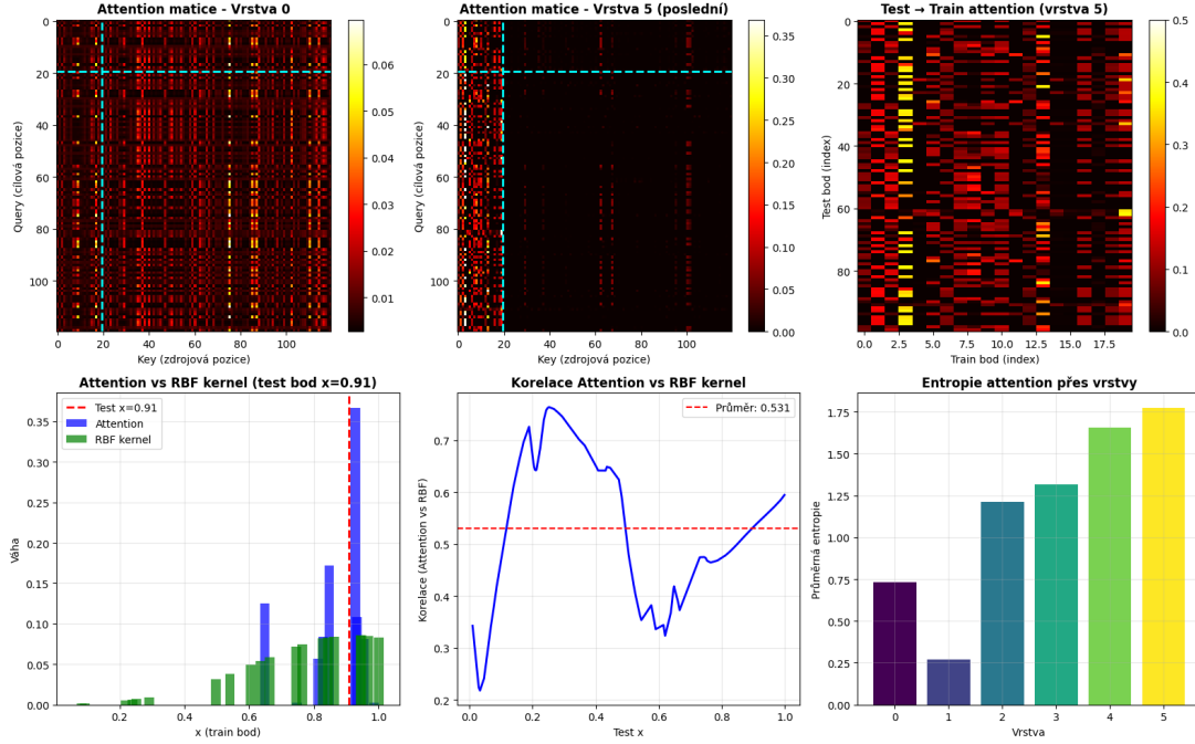
Obrázek 3.2: Detail attention vah poslední vrstvy (průměr přes 8 hlav) pro vybraný testovací bod v porovnání s normalizovanými RBF vahami. Attention je výrazně ostřejší, koncentruje téměř veškerou váhu na nejbližší bod, zatímco RBF distribuuje váhu plynule.
