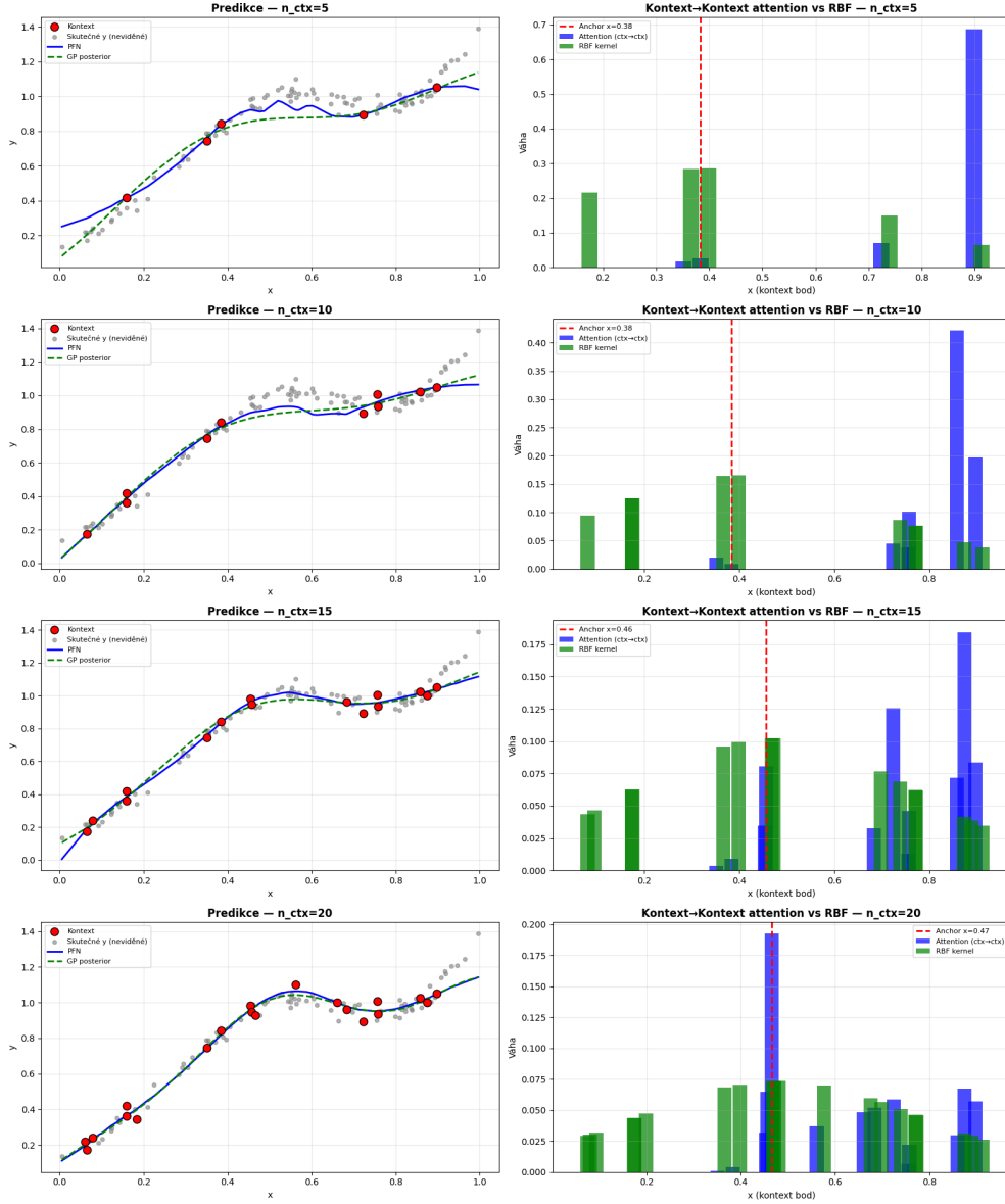
Obrázek 3.4: 100-epoch model: vizualizace predikcí pro n \in \{5, 10, 15, 20\} . Červené body: kontextová data dostupná modelu; šedé body: skutečné neviděné hodnoty; modrá: PFN; zelená přerušovaná: GP posterior se správným \ell . Všechny řádky vychází ze stejné GP realizace, liší se pouze velikostí kontextu. Od n = 15 obě křivky téměř splývají.
