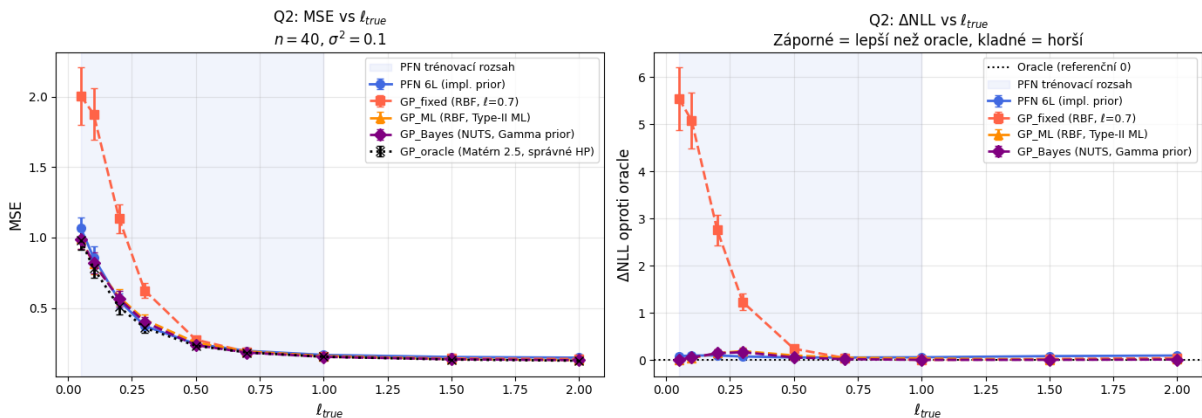
Obrázek 3.20: Vliv síly misspecifikace ( n = 40 ). Vlevo: MSE jako funkce \ell_{\text{true}} . Vpravo: \Delta\text{NLL} vůči oracle . Modrý pás značí trénovací rozsah PFN \ell \in [0,05, 1,0] . GP_fixed (oranžová) pro krátké korelační délky selhává v obou metrikách, ostatní metody se s rostoucím \ell_{\text{true}} sbíhají k oracle . PFN zůstává blízko oracle v celém rozsahu včetně hodnot mimo svůj trénovací rozsah.
