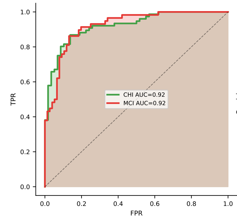
ROC-AUC
