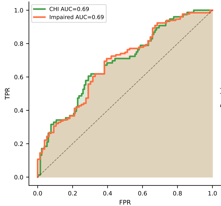
ROC-AUC
