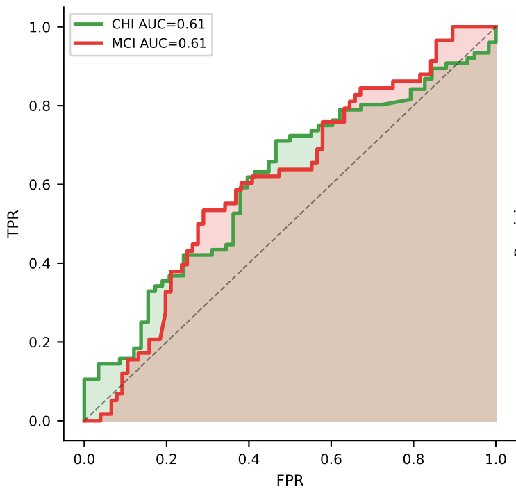
ROC-AUC
