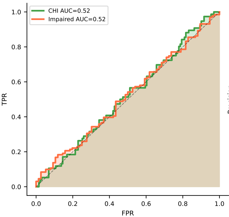
ROC-AUC
