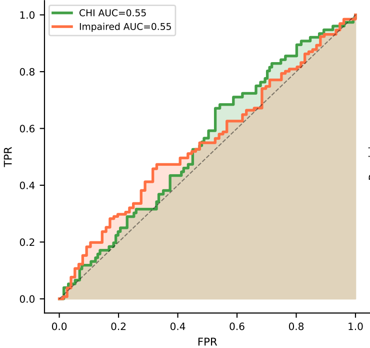
ROC-AUC
