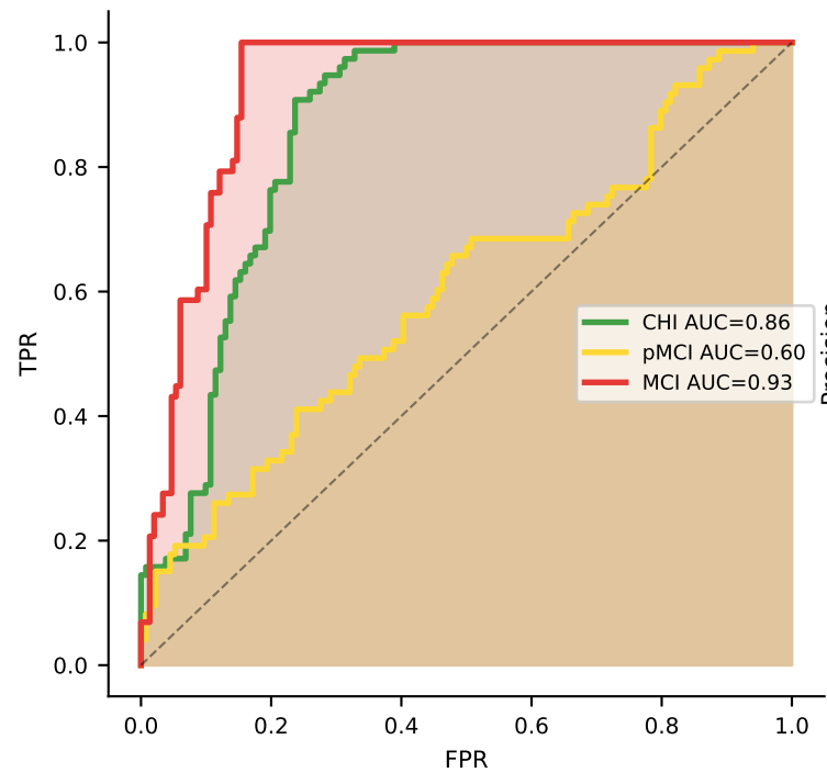
ROC-AUC
