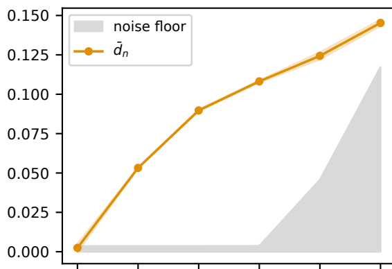
IAAFT
