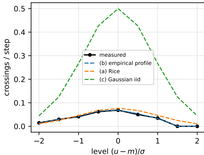
SC2 keyword spotting, h1 ch27 (kurt 2.7)
