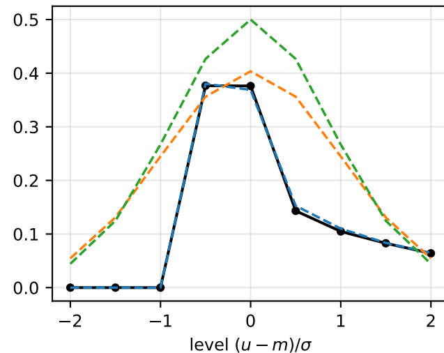
enwik8 char-LM, l0.fc2_in ch473 (kurt 389.4)
