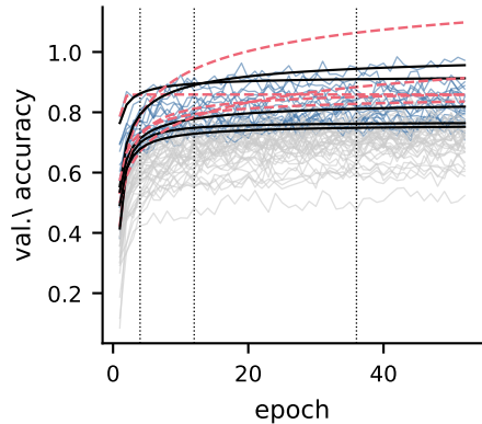
(a) SH survivors, naive fits (--) vs true curves (—)
