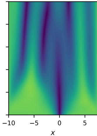
vanilla PINN
