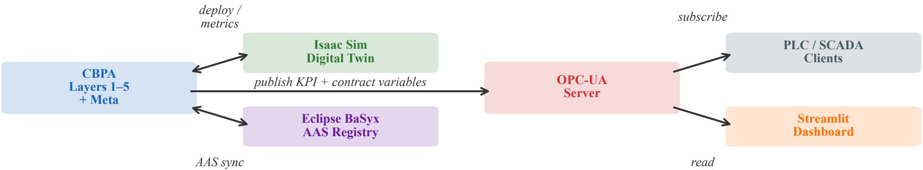
(d) Integrated execution stack data flow
