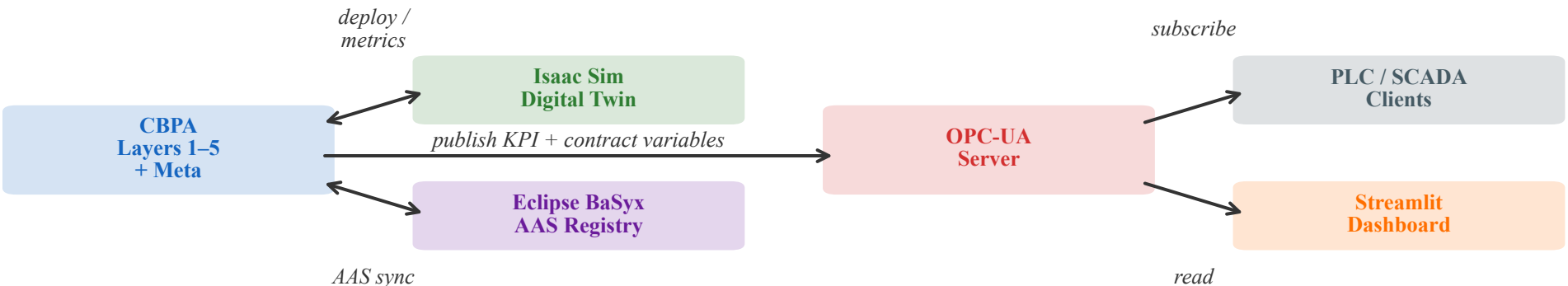
(d) Integrated execution stack data flow
